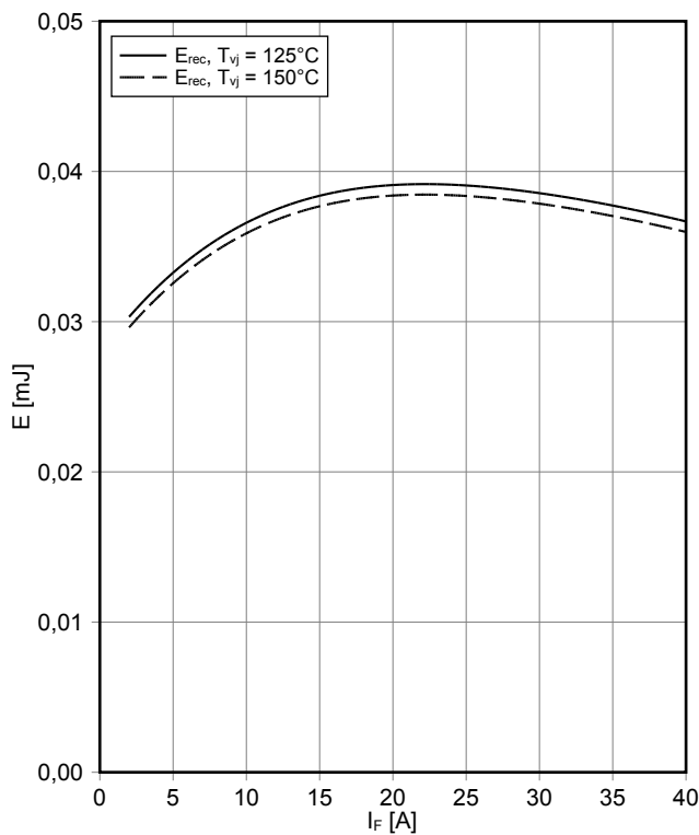
スイッチング損失 Diode, アップコンバータ (Typical) switching losses Diode, Boost (typical) E_{rec} = f(I_F) R_{Gon} = 2.7 \Omega, V_{CE} = 400 V
