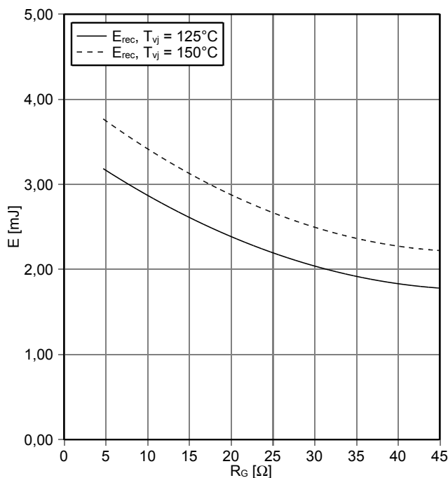
Schaltverluste Diode-Chopper (typisch) switching losses Diode-Chopper (typical) E_{rec} = f(R_G) I_F = 30 \text{ A} , V_{CE} = 600 \text{ V}
