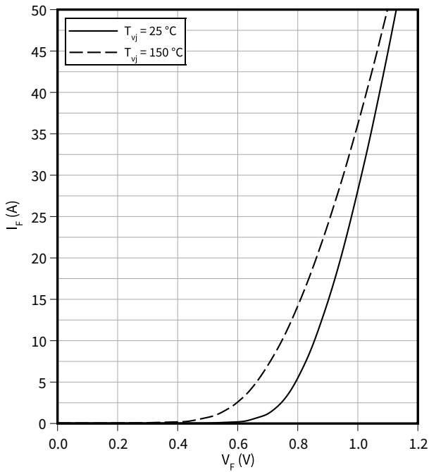
Durchlasskennlinie (typisch), Verpolschutz Diode B
