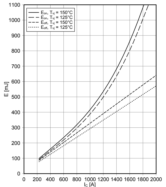
スイッチング損失 IGBT-ブレーキチョッパー (Typical) switching losses IGBT, Brake-Chopper (typical) E_{on} = f(I_C) , E_{off} = f(I_C) V_{GE} = \pm 15\text{ V} , R_{Gon} = 1.2\ \Omega , R_{Goff} = 1.8\ \Omega , V_{CE} = 900\text{ V}
