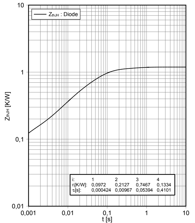
過渡熱インピーダンス Diode、ブレーキチョッパー transient thermal impedance Diode, Brake-Chopper Z_{thJH} = f(t)
