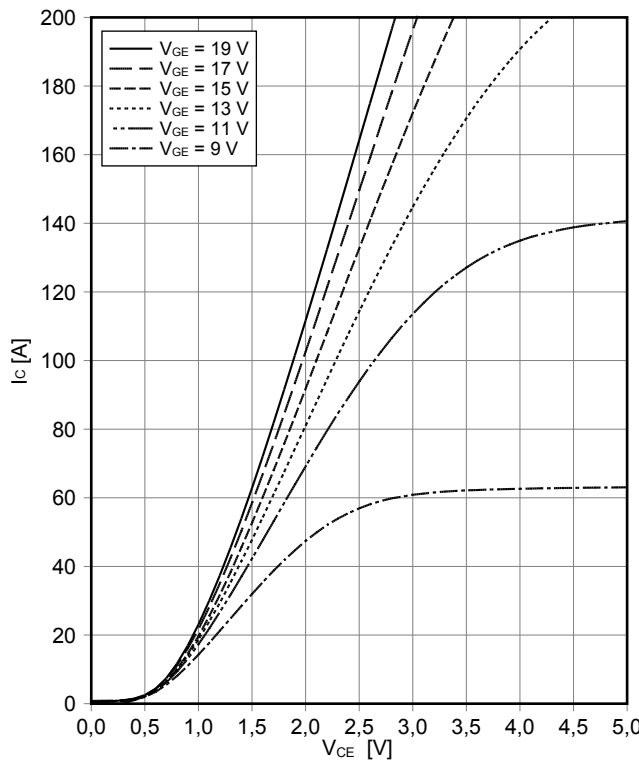
出力特性 IGBT-ブレーキチョッパー (Typical) output characteristic IGBT, Brake-Chopper (typical) I_C = f(V_{CE}) T_{vj} = 150^\circ\text{C}
