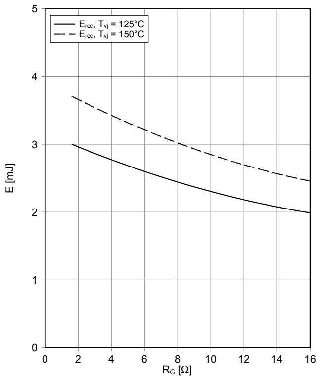
スイッチング損失 Diode、ブレーキチョッパー (Typical) switching losses Diode, Brake-Chopper (typical) E_{rec} = f(R_G) I_F = 50 \text{ A}, V_{CE} = 600 \text{ V}
