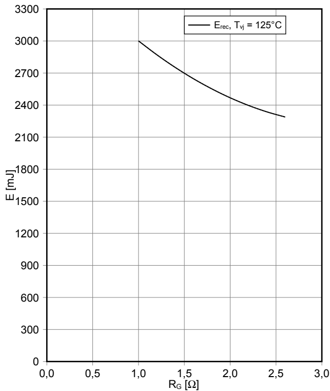
スイッチング損失 Diode、インバータ (Typical) switching losses Diode, Inverter (typical) E_{rec} = f(R_G) I_F = 750\text{ A}, V_{CE} = 3600\text{ V}
