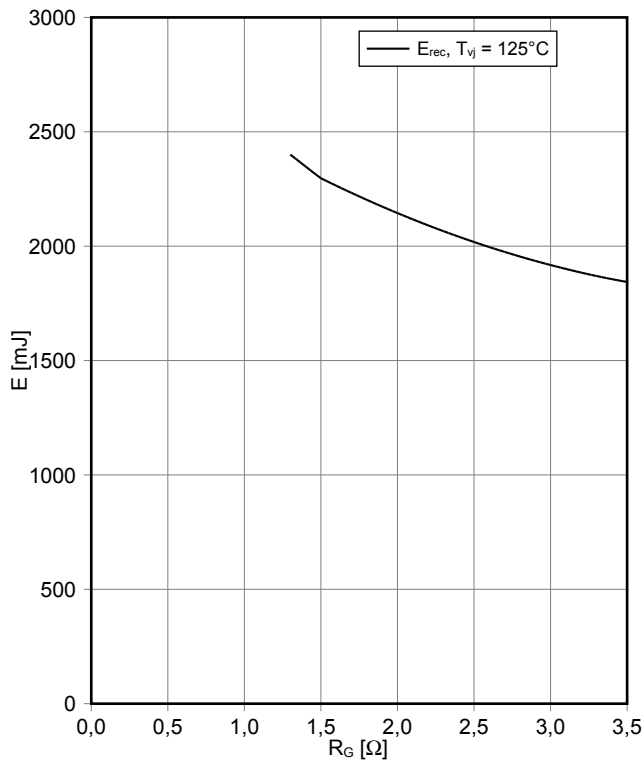
スイッチング損失 Diode、インバータ (Typical) switching losses Diode, Inverter (typical) E_{rec} = f(R_G) I_F = 600 \text{ A}, V_{CE} = 3600 \text{ V}
