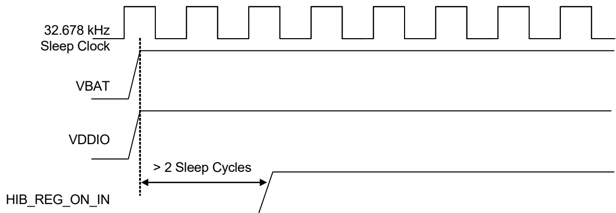
Figure 38. HIB_REG_ON_IN = High, HIB_REG_ON_OUT Connected to REG_ON
