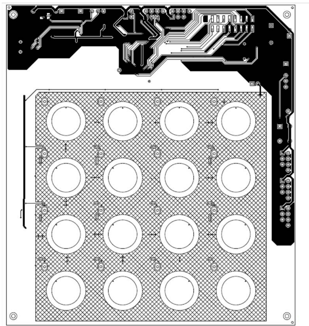
Figure 18. Top Layer
