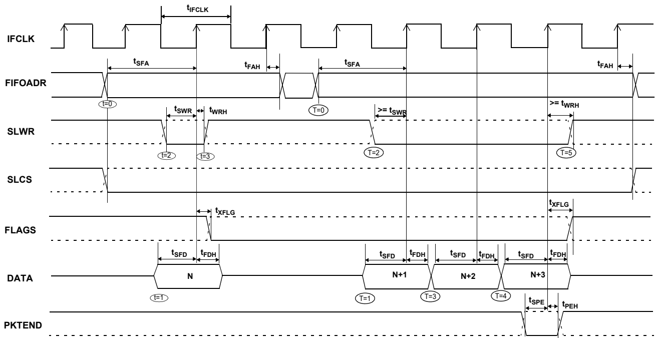
图 32. 从器件 FIFO 同步写入序列和时序图 [52]
