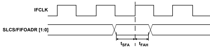
图 28. 从器件 FIFO 同步地址时序图 [48]
