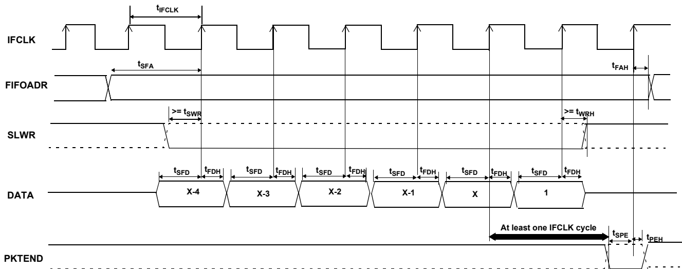
图 24. 从器件 FIFO 同步写入序列和时序图 [46]
