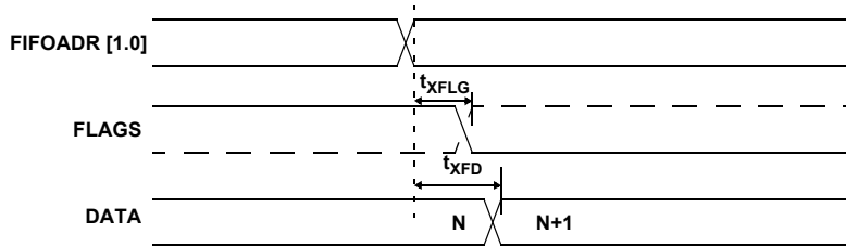
图 27. 从器件 FIFO 标志 / 数据时序图寻址 [48]
