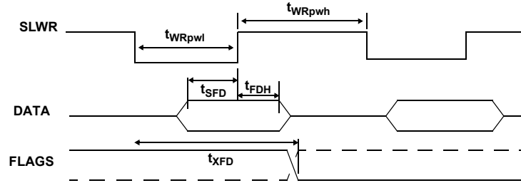
图 22. 从器件 FIFO 异步写入时序图 [42]
