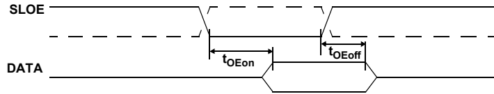
图 26. 从器件 FIFO 输出使能时序图 [48]
