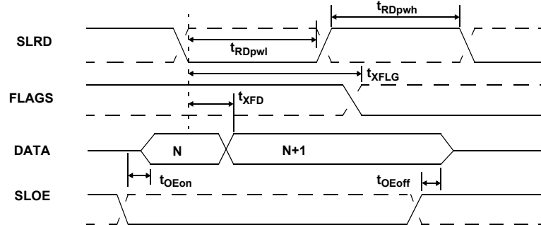
图 20. 从器件 FIFO 异步读取时序图 [38]
