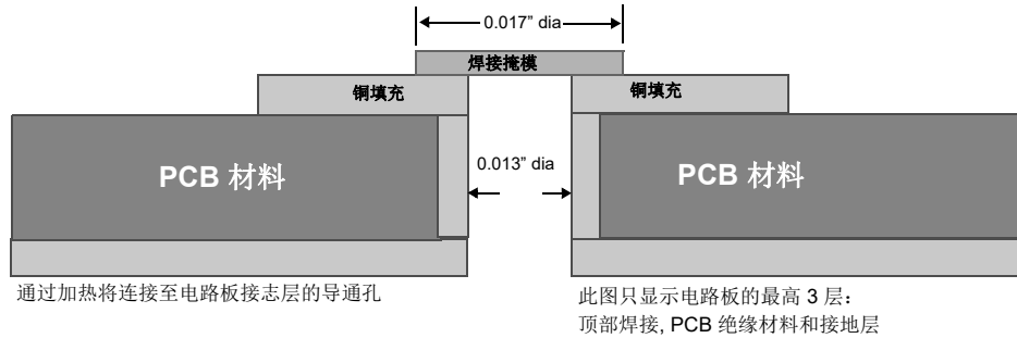
图 41. QFN 封装底部区域的横截面
