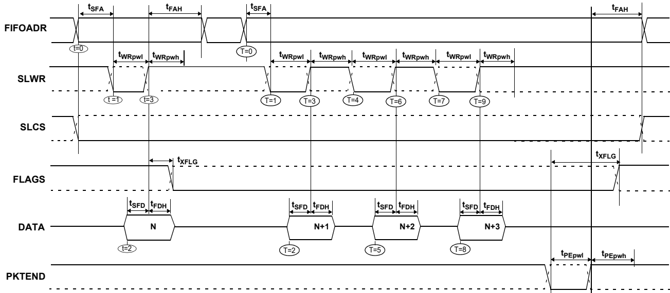
图 35. 从器件 FIFO 异步写入序列和时序图 [54]
