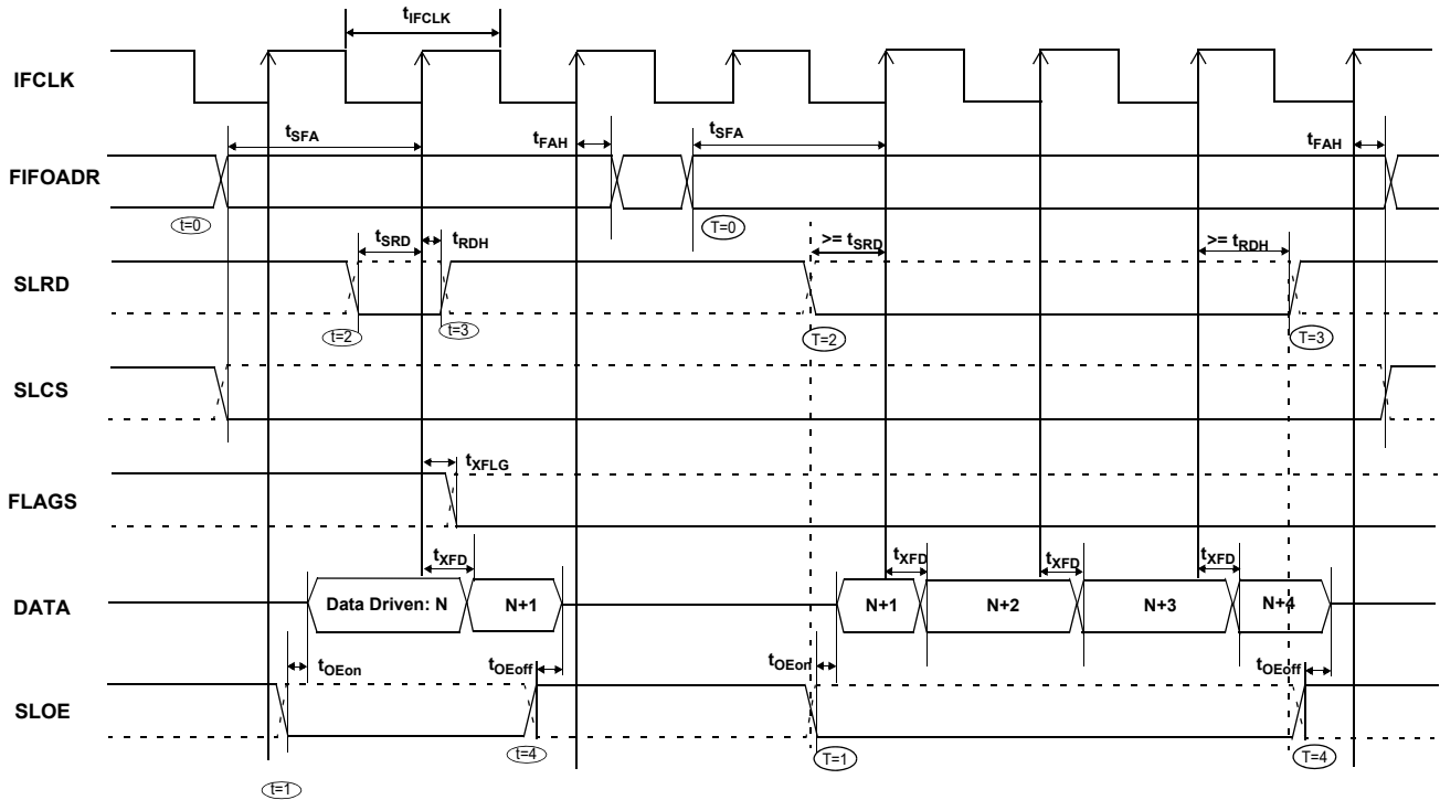
图 30. 从器件 FIFO 同步读取序列和时序图 [50]
