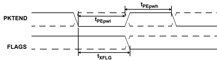
图 25. 从器件 FIFO 异步数据包结束探针时序图 [46]
