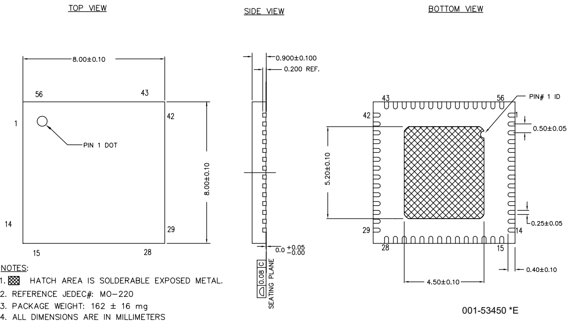
图 37. 56 引脚 QFN 8 × 8 mm Sawn 版本 (001-53450)
