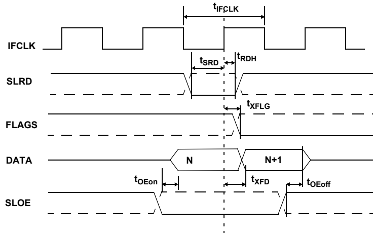
图 19. 从器件 FIFO 同步读取时序图 [36]
