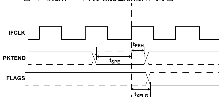
图 23. 从器件 FIFO 同步数据包结束探针时序图 [44]
