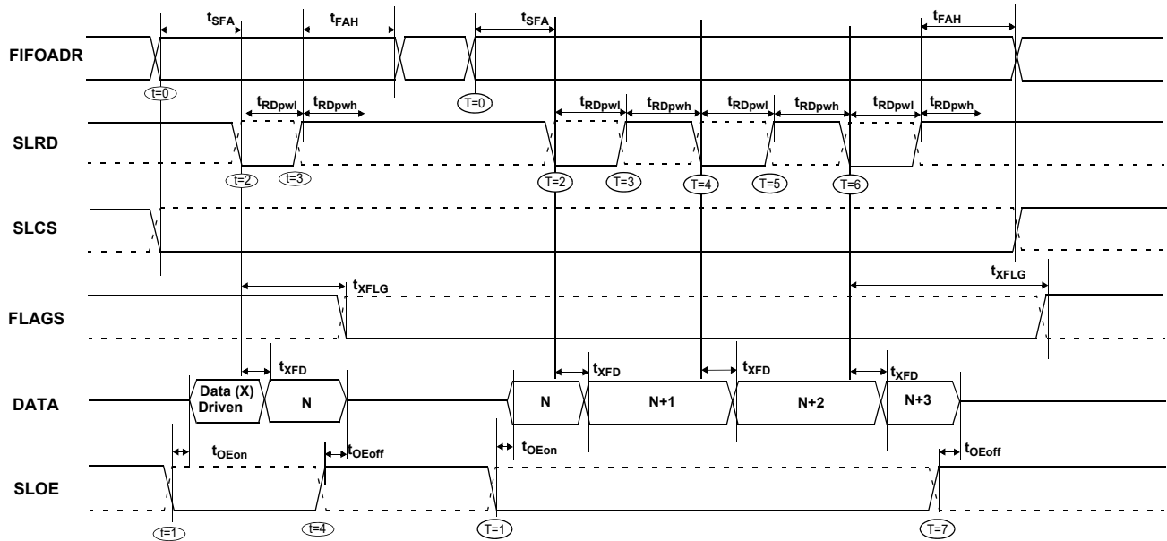
图 33. 从器件 FIFO 异步读取序列和时序图 [53]
