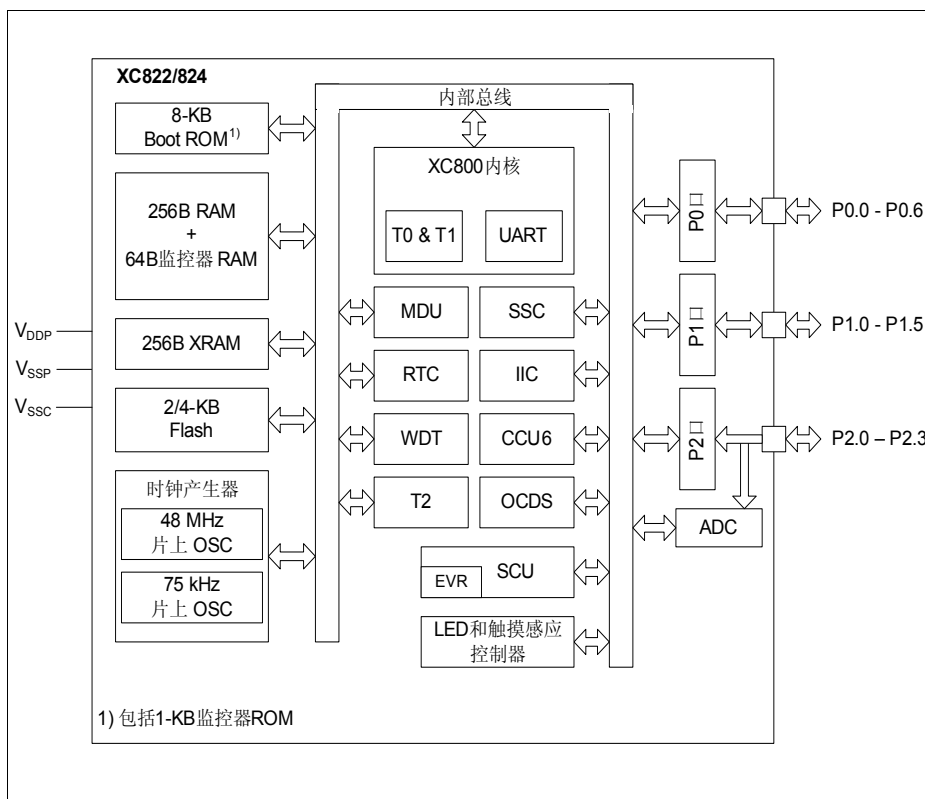
图 2 XC822/824 框图
