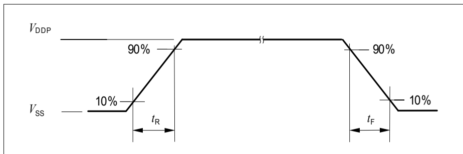
图 12 上升 / 下降时间参数
