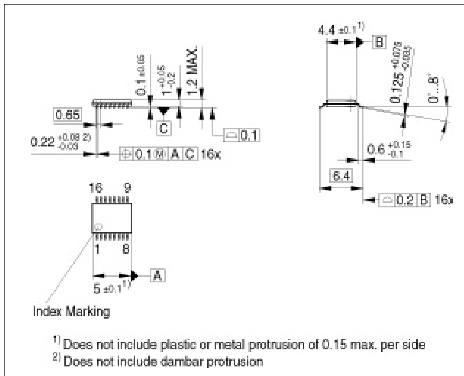
图 18 PG-TSSOP-16-1 封装图
