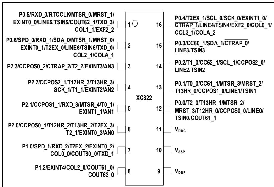
图 4 XC822 引脚配置，PG-TSSOP-16 封装（顶视图）
