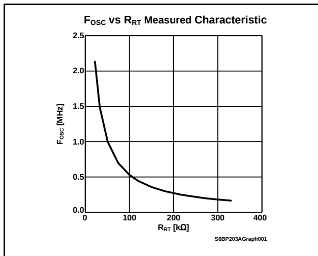
Figure 9-1 F OSC vs R RT の実測特性
