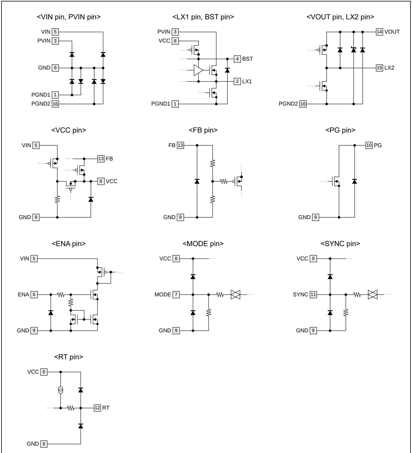
Figure 3-1 入出力端子等価回路図
