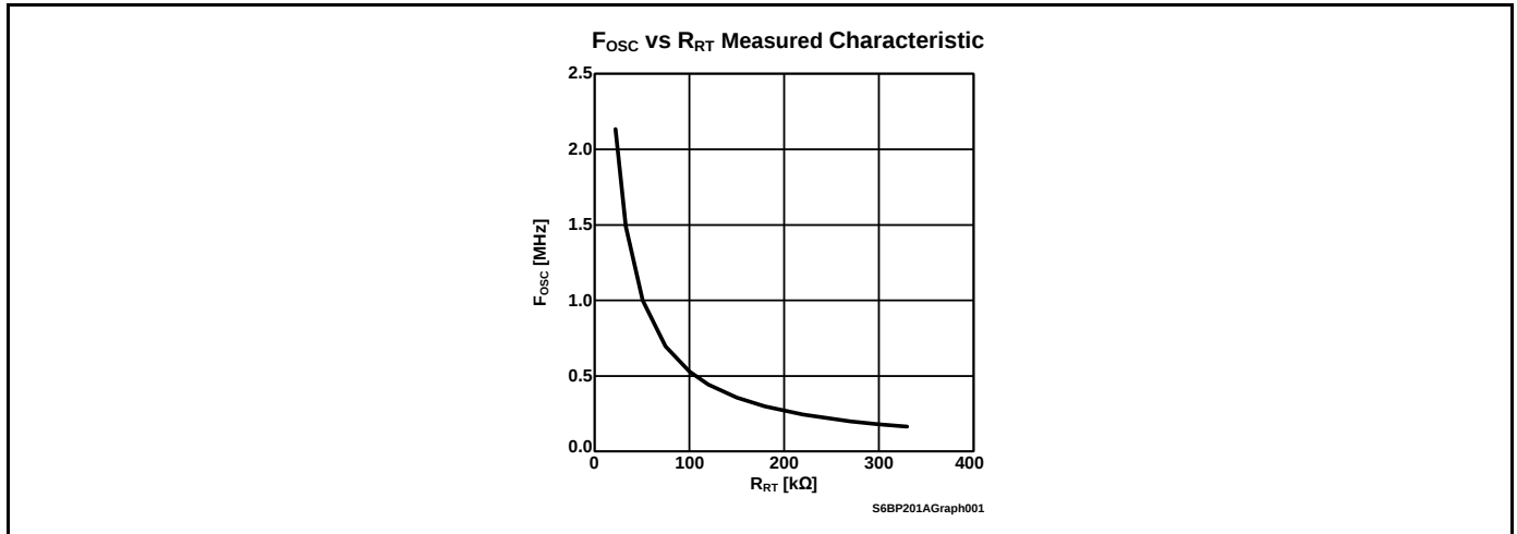
Figure 10-1 F OSC vs R RT の実測特性
