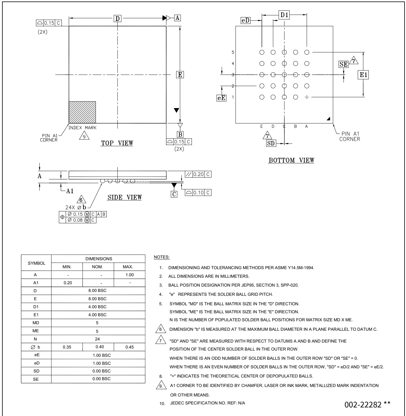
Figure 65 24 ボール BGA (8 × 8 × 1 mm) VAC024 パッケージ外形 (PG-BGA-24), 002-22282
