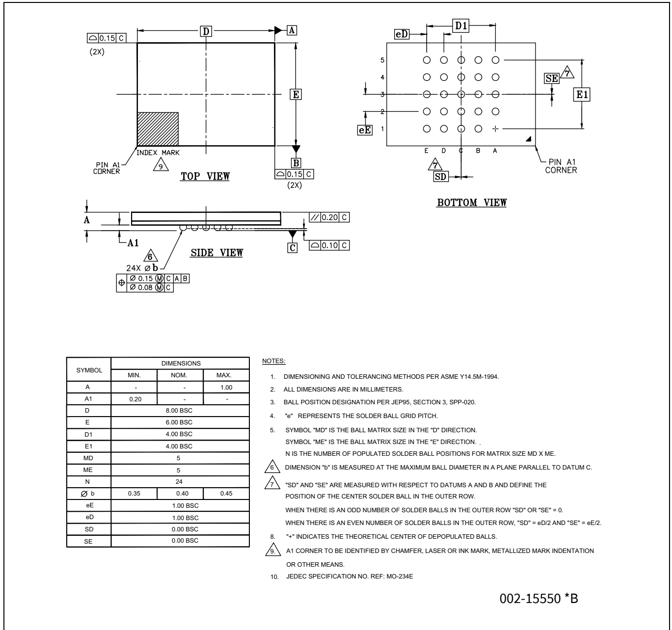
Figure 64 24 ボール BGA (8 × 6 × 1mm) VAA024/ELA024/E2A024 パッケージ外形 (PG-BGA-24), 002-15550
