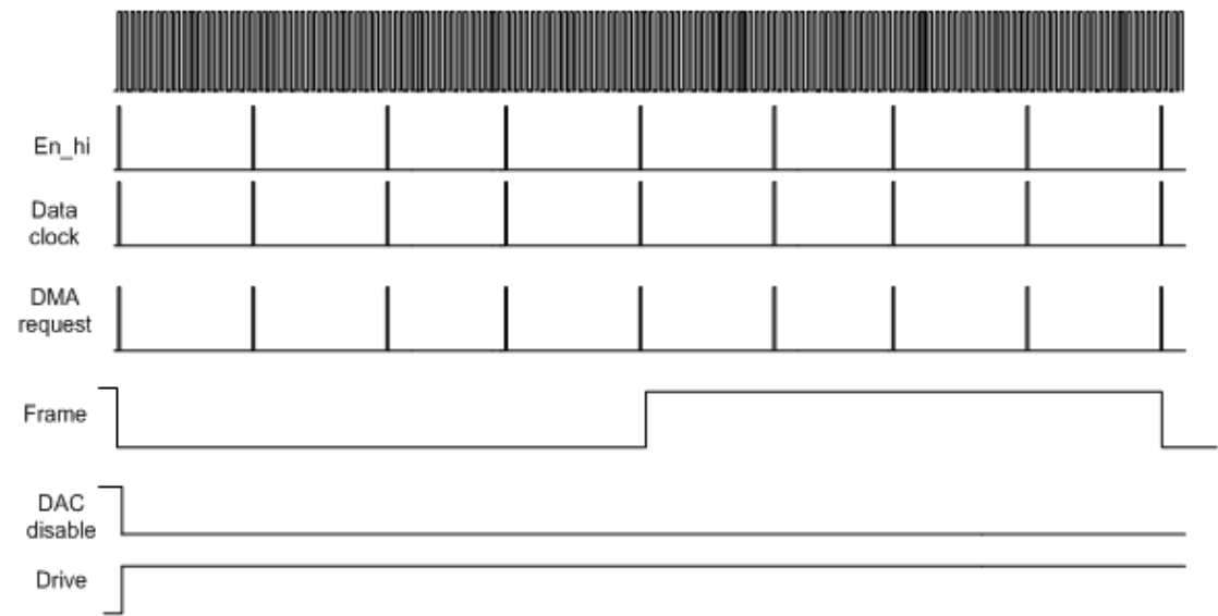
图 2. 段显示器控制信号类型 B 波形（始终运行模式）
