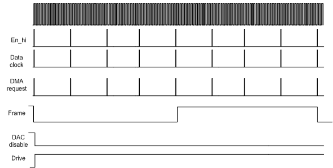
图 2. 段显示器控制信号类型 B 波形（始终为有效模式）
