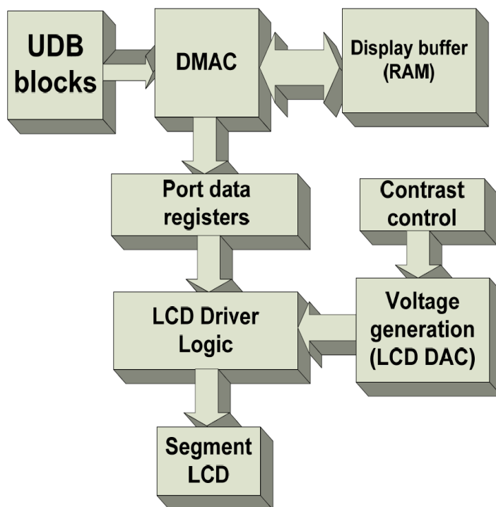
图 7. 高级段显示器
