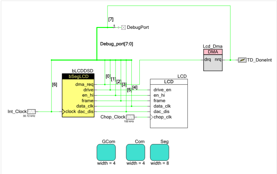
图 6. 段显示器组件原理图
