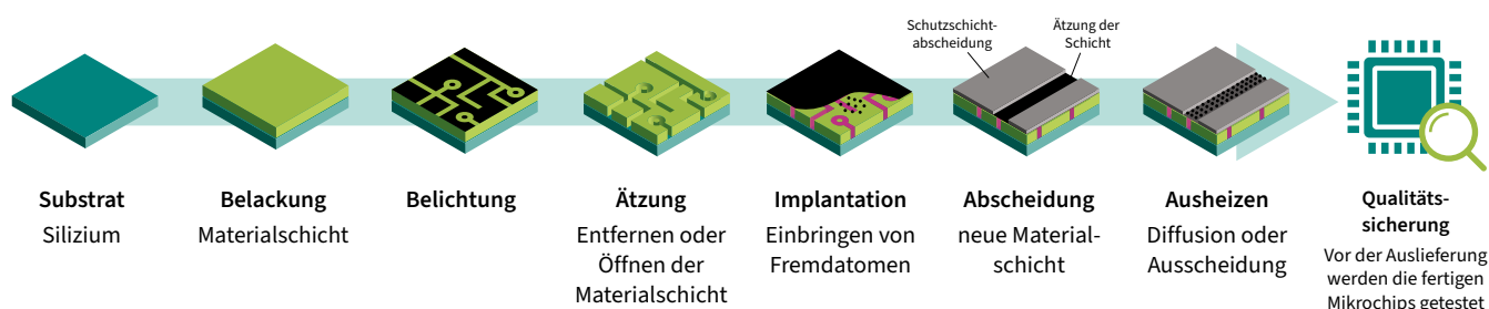
Halbleiterprozessierung: schematische Prozessschritte Wiederkehrende Arbeitsschritte je nach Chip
