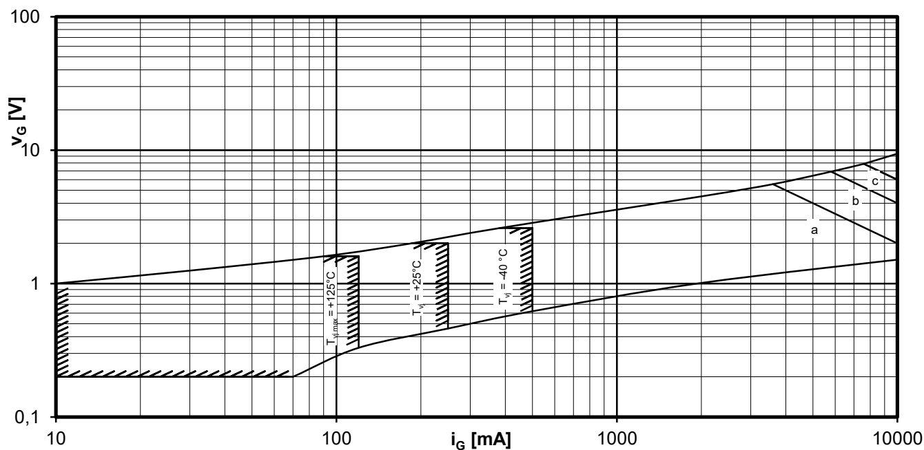
Steuercharakteristik v_G = f(i_G) mit Zündbereichen für V_D = 12\text{ V} Gate characteristic v_G = f(i_G) with triggering area for V_D = 12\text{ V}
