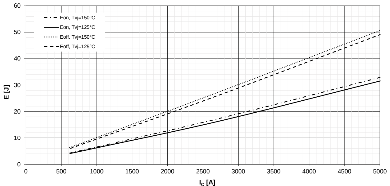
Schaltverluste IGBT, Wechselrichter (typisch) switching losses IGBT, Inverter (typical)
