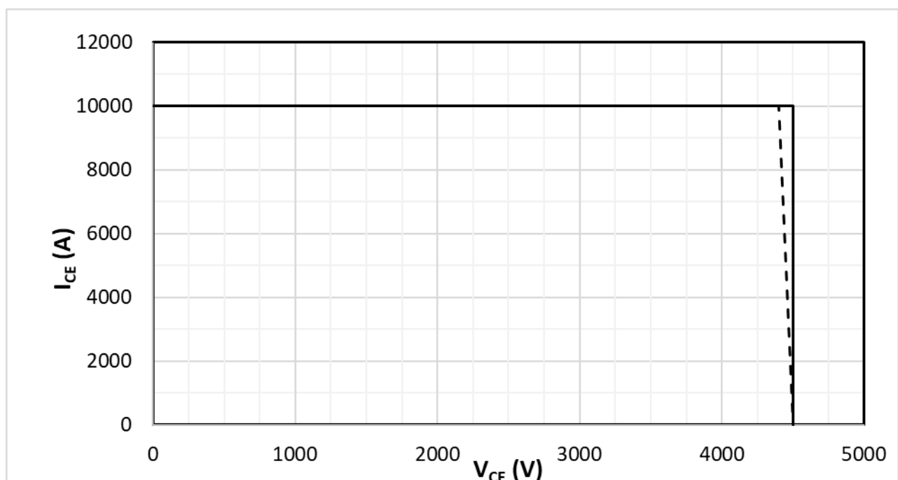
Sicherer Rückwärts-Arbeitsbereich IGBT, Wechselrichter (RBSOA) Reverse bias safe operating area IGBT, Inverter (RBSOA)
