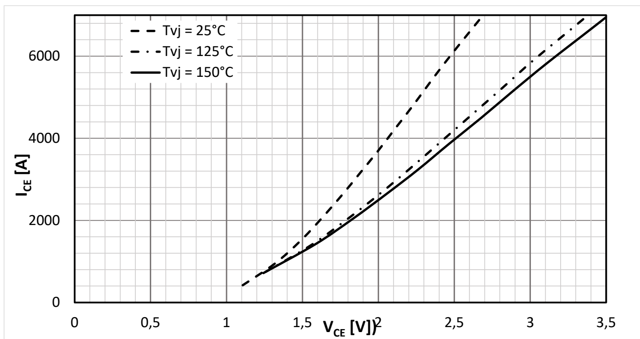
Ausgangskennlinie IGBT, Wechselrichter (typisch) output characteristic IGBT, Inverter (typical)
