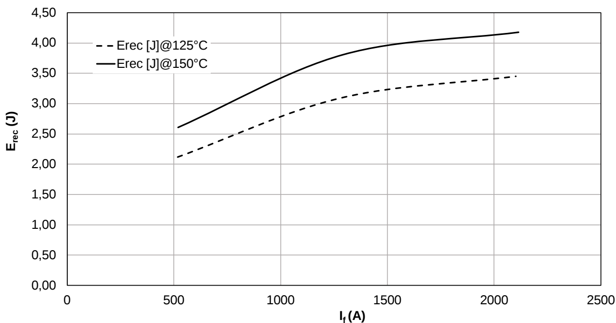
Schaltverluste Diode, Wechselrichter (typisch) switching losses Diode, Inverter (typical) E_{rec}=f(I_F) R_{Gon}=1.0\Omega , V_{CE}=2800\text{V}
