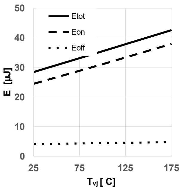
图 15 典型开关能量损耗随结温变化关系
