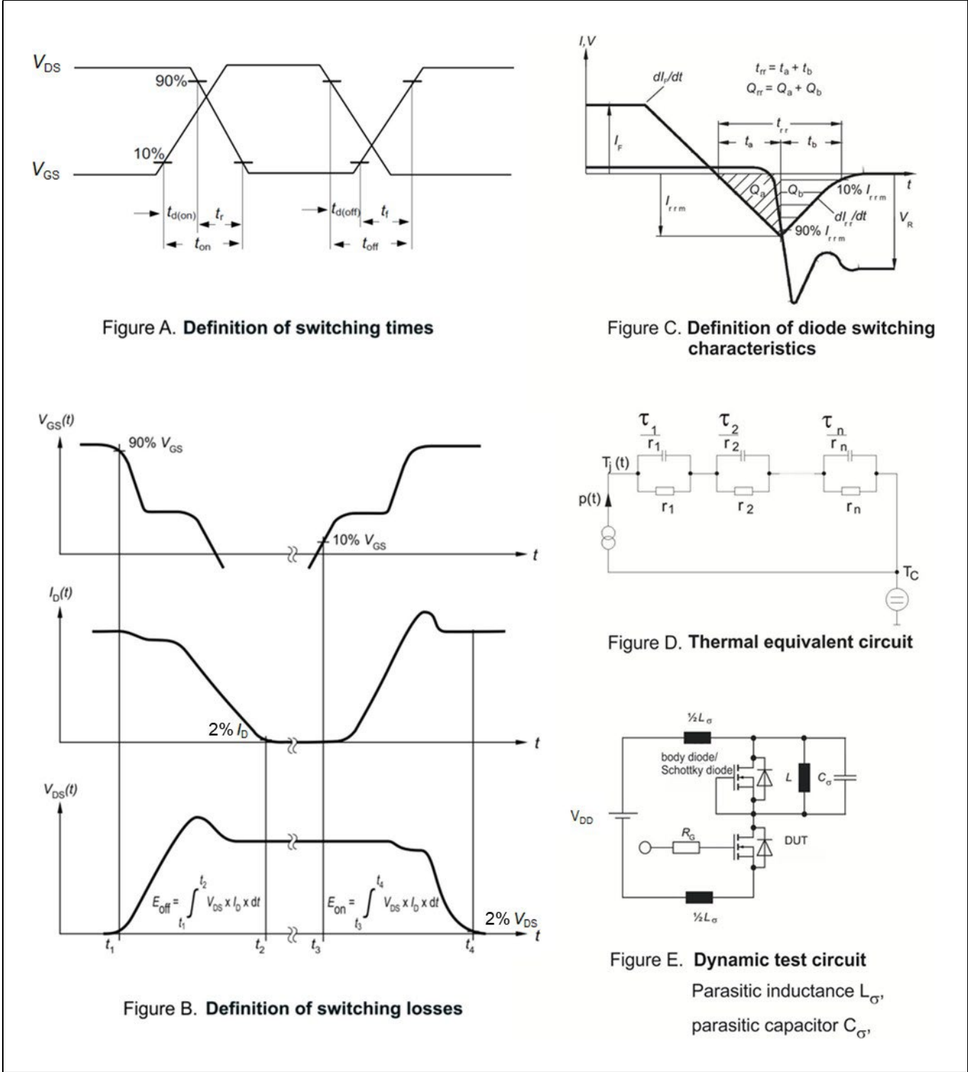
图 23 测试条件
