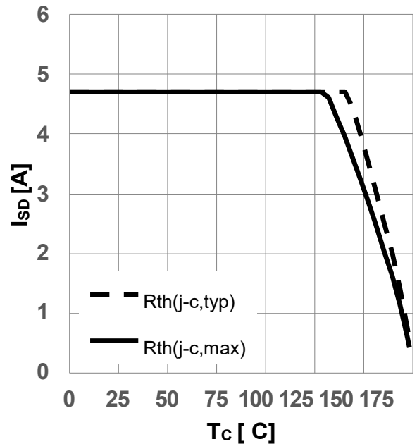
图 4 最大源漏电流随壳温 (受限于接合线) 变化关系 ( I_{SD} = f(T_C) , V_{GS} = 0V )
