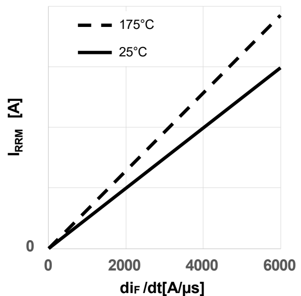
图 20 典型反向恢复电流随二极管电流斜率变化关系 (I_{rrm} = f(di_F/dt), V_{DD} = 800V, V_{GS} = 0V/18V, I_D = 2A, \text{独立负载, 测试电路如图 E 所示, 体二极管在 } V_{GS} = 0V \text{ 时})
