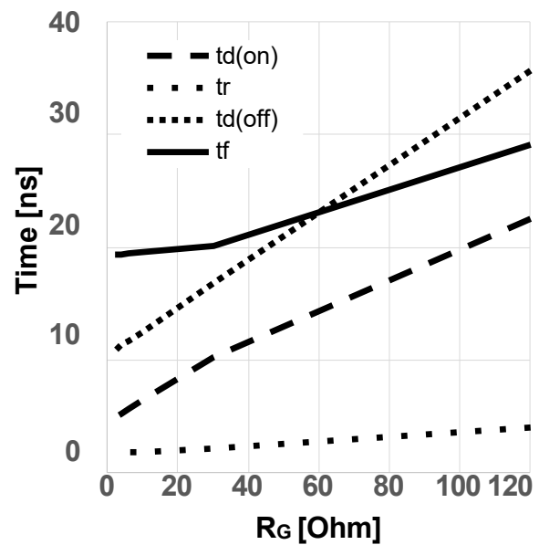
图 18 典型开关时间随栅极电阻变化关系 (t = f(R_{G,ext}), V_{DD} = 800V, V_{GS} = 0V/18V, I_D = 2A, T_{vj} = 175^\circ C, \text{独立负载, 测试电路见图 E, 二极管: } V_{GS} = 0V \text{ 时的体二极管})
