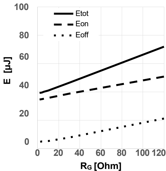
图 17 典型开关能量损耗随栅极电阻变化关系 (E = f(R_{G,ext}), V_{DD} = 800V, V_{GS} = 0V/18V, I_D = 2A, T_{vj} = 175^\circ C, \text{独立负载, 测试电路见图 E, 二极管: } V_{GS} = 0V \text{ 时的体二极管})
