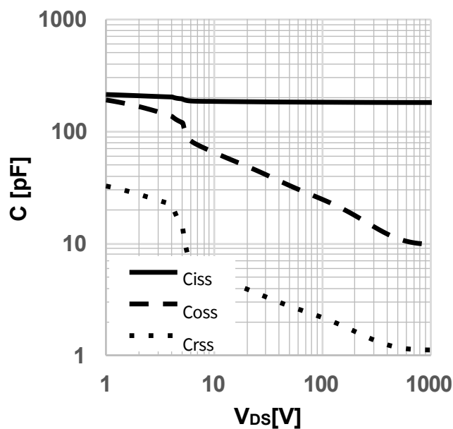
图 11 典型电容随漏源电压变化关系
