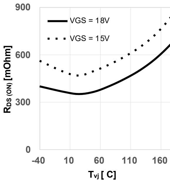
图 9 典型导通电阻随结温变化关系
