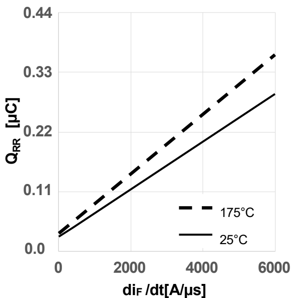
图 19 典型的反向恢复电荷随二极管电流斜率变化关系 (Q_{rr} = f(di_F/dt), V_{DD} = 800V, V_{GS} = 0V/18V, I_D = 2A, \text{独立负载, 测试电路见图 E, } V_{GS} = 0V \text{ 时的体二极管})
