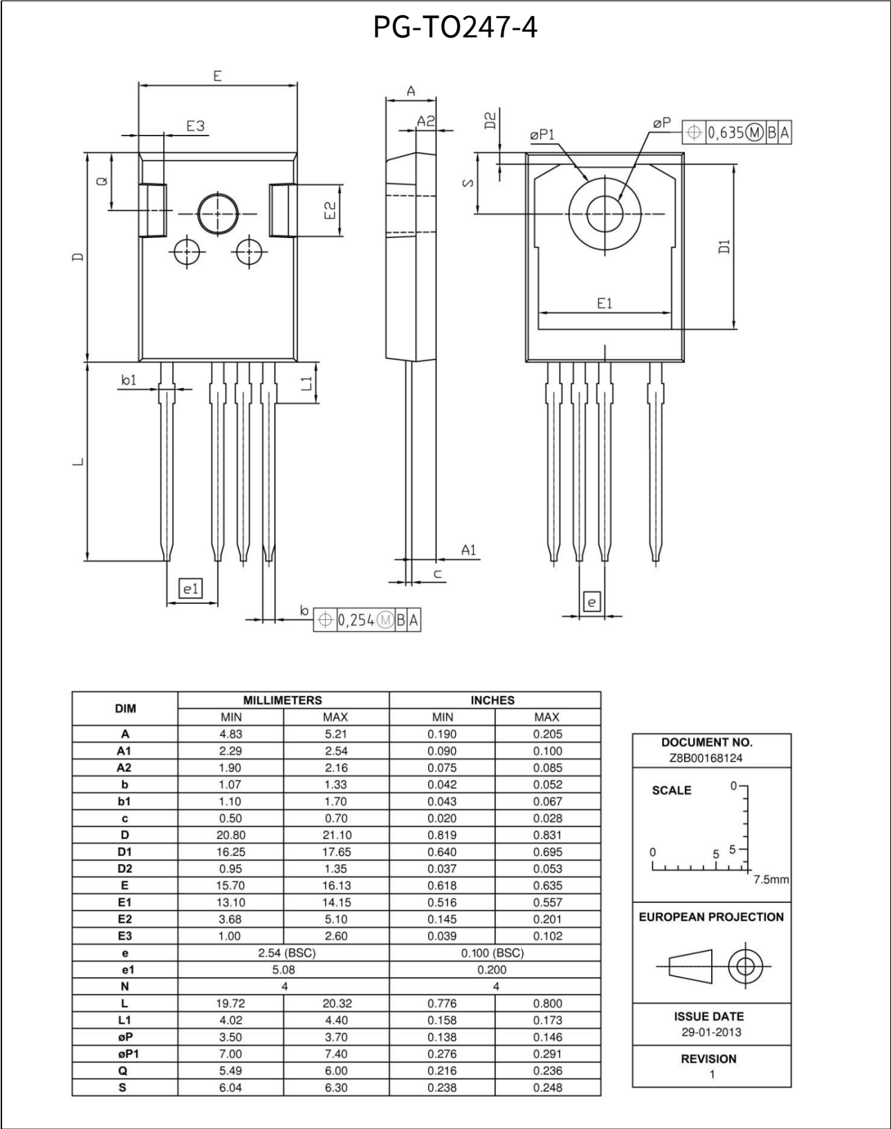
图 22 封装图
