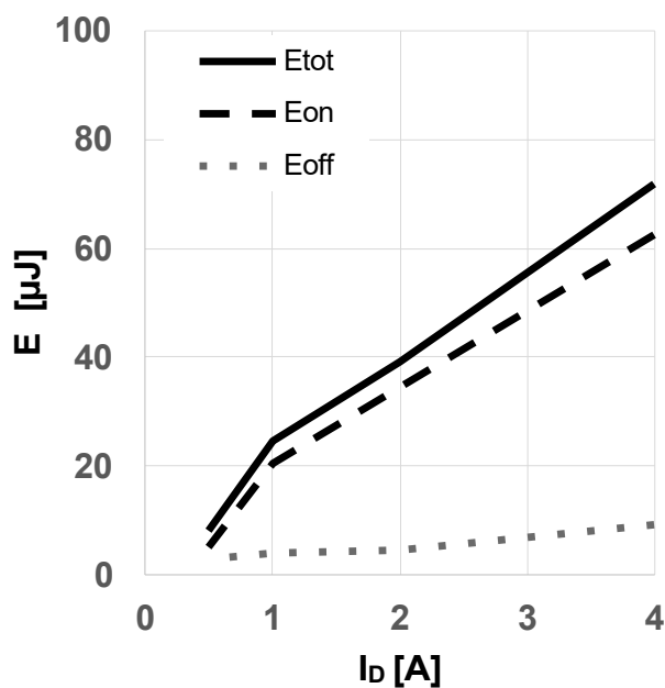
图 16 典型开关能量损耗随漏源电流变化关系
