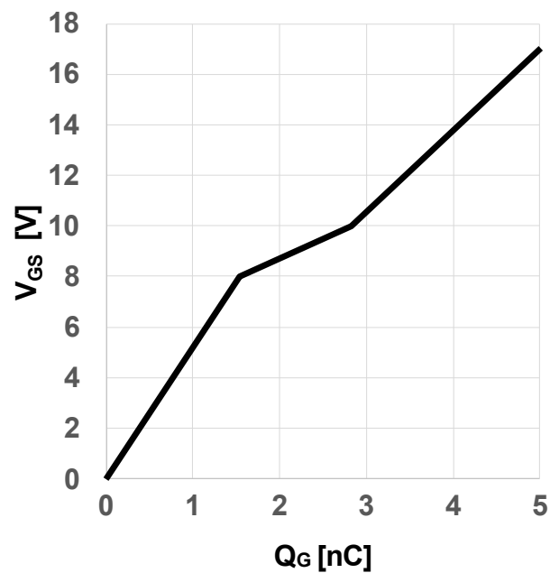
图 10 典型栅极电荷
