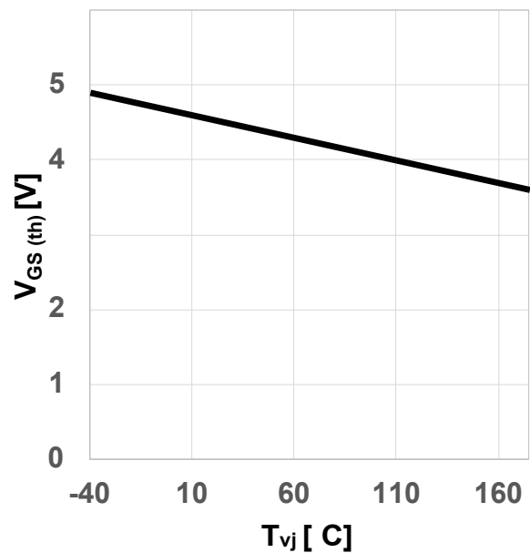
图 6 典型栅极-源极阈值电压与结温的函数关系
