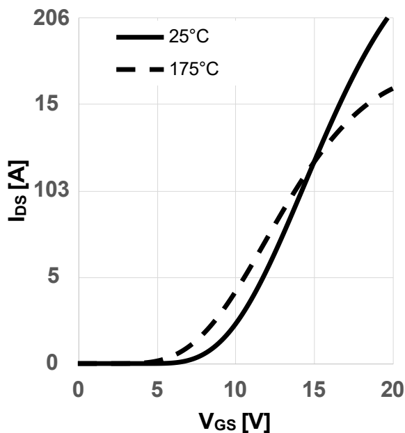
图 5 典型传输特性
