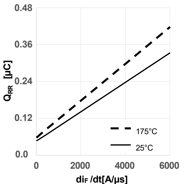
图 19 典型的反向恢复电荷随二极管电流斜率变化关系 (Q_{rr} = f(di_f/dt), V_{DD} = 800V, V_{GS} = 0V/18V, I_D = 4A, \text{独立负载, 测试电路见图 E, } V_{GS} = 0V \text{ 时的体二极管})
