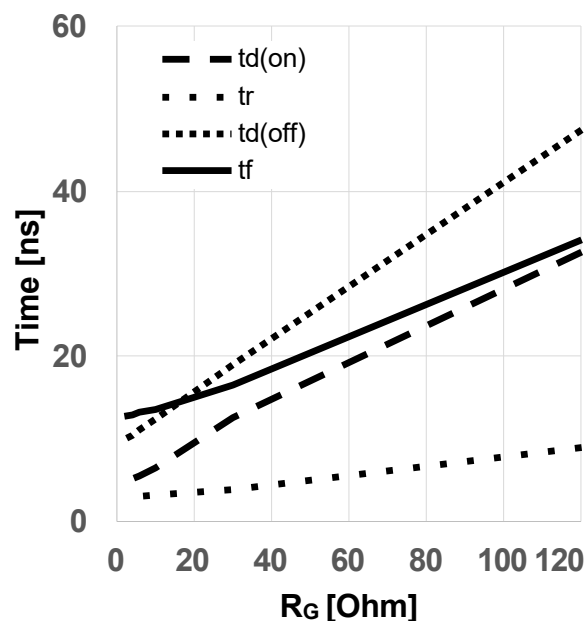
图 18 典型开关时间随栅极电阻变化关系 (t = f(R_{G,ext}), V_{DD} = 800V, V_{GS} = 0V/18V, I_D = 4A, T_{vj} = 175^\circ C, \text{独立负载, 测试电路见图 E, 二极管: } V_{GS} = 0V \text{ 时的体二极管})
