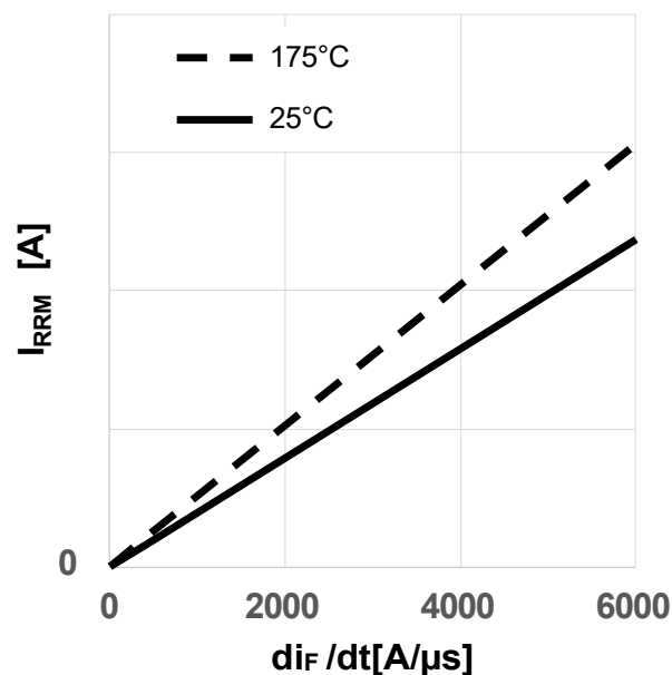
图 20 典型反向恢复电流随二极管电流斜率变化关系 (I_{rrm} = f(di_f/dt), V_{DD} = 800V, V_{GS} = 0V/18V, I_D = 4A, \text{独立负载, 测试电路如图 E 所示, 体二极管在 } V_{GS} = 0V \text{ 时})
