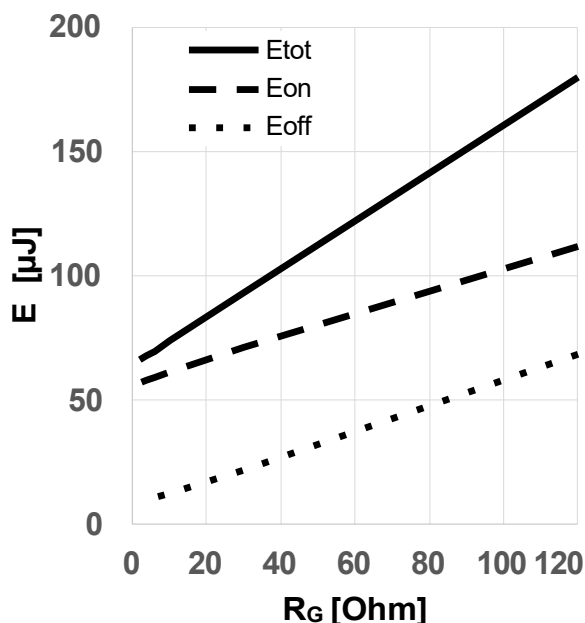
图 17 典型开关能量损耗随栅极电阻变化关系 (E = f(R_{G,ext}), V_{DD} = 800V, V_{GS} = 0V/18V, I_D = 4A, T_{vj} = 175^\circ C, \text{独立负载, 测试电路见图 E, 二极管: } V_{GS} = 0V \text{ 时的体二极管})
