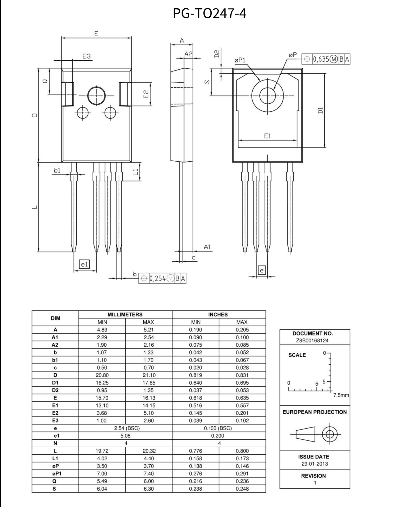
图 22 封装图
