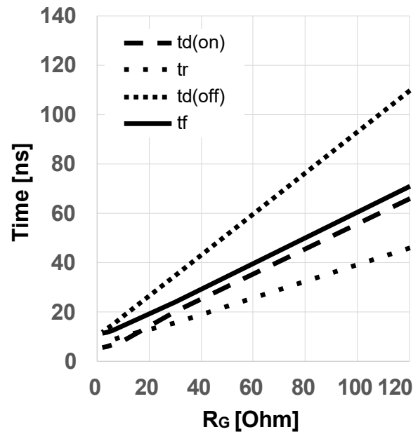
图 18 典型开关时间随栅极电阻变化关系 (t = f(R_{G,ext}), V_{DD} = 800V, V_{GS} = 0V/18V, I_D = 8.5A, T_{vj} = 175^\circ C, \text{独立负载, 测试电路见图 E, 二极管: } V_{GS} = 0V) \text{ 时的体二极管}
