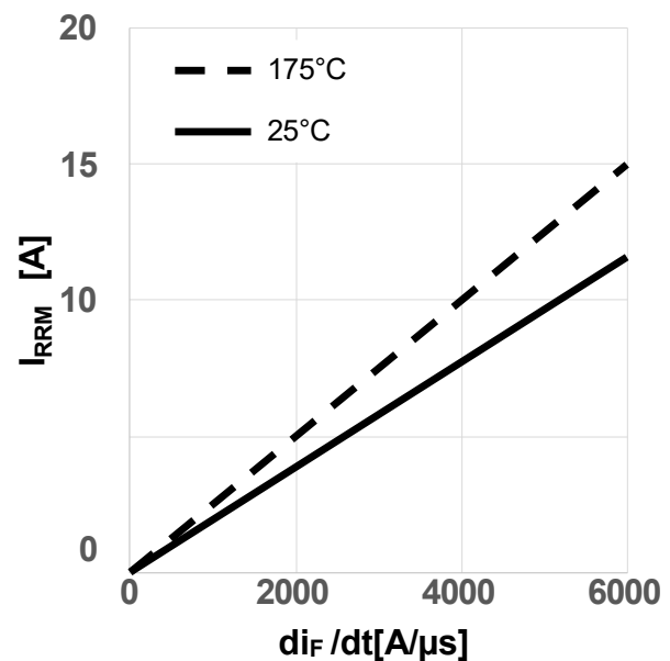
图 20 典型反向恢复电流随二极管电流斜率变化关系 (I_{rrm} = f(di_i/dt), V_{DD} = 800V, V_{GS} = 0V/18V, I_D = 8.5A, \text{独立负载, 测试电路如图 E 所示, 体二极管在 } V_{GS} = 0V \text{ 时})
