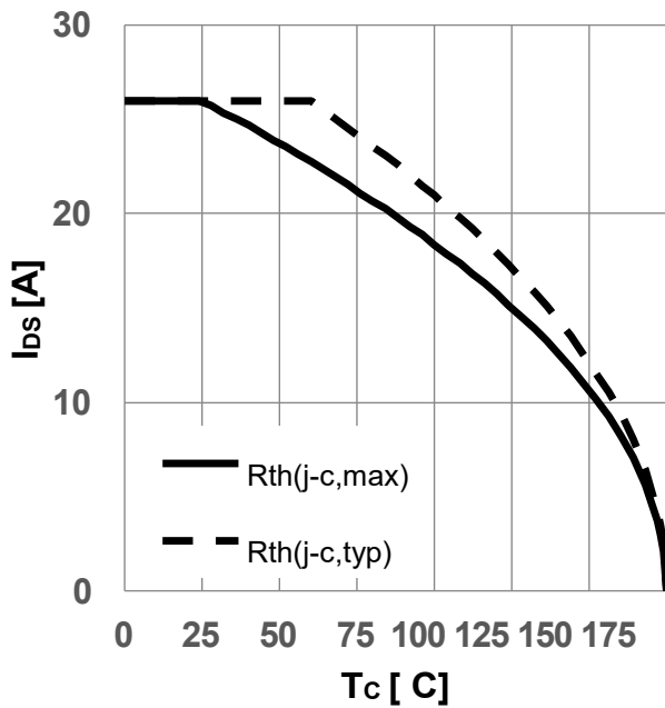
图 3 最大直流漏源电流随壳温 (受限于 接合线) 变化关系 ( I_{DS} = f(T_c) )
