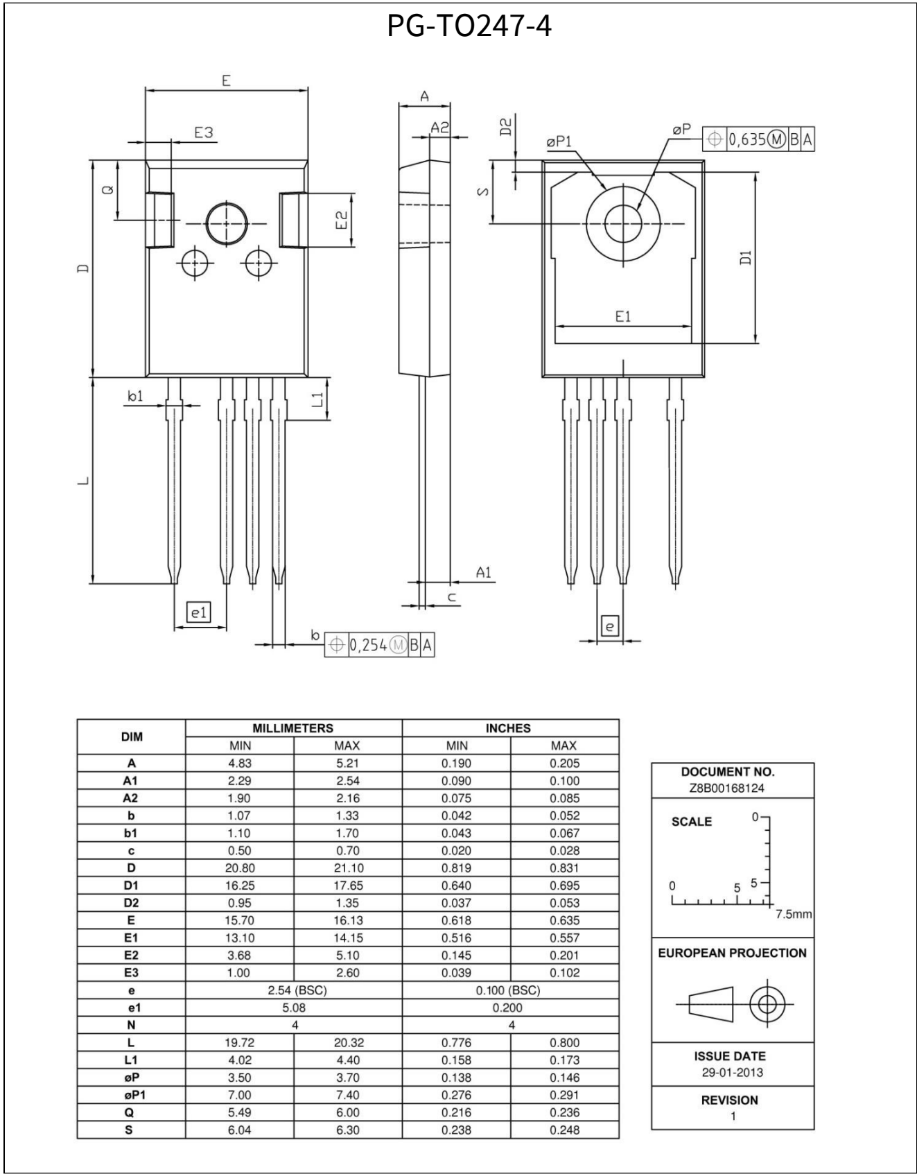
图 22 封装图
