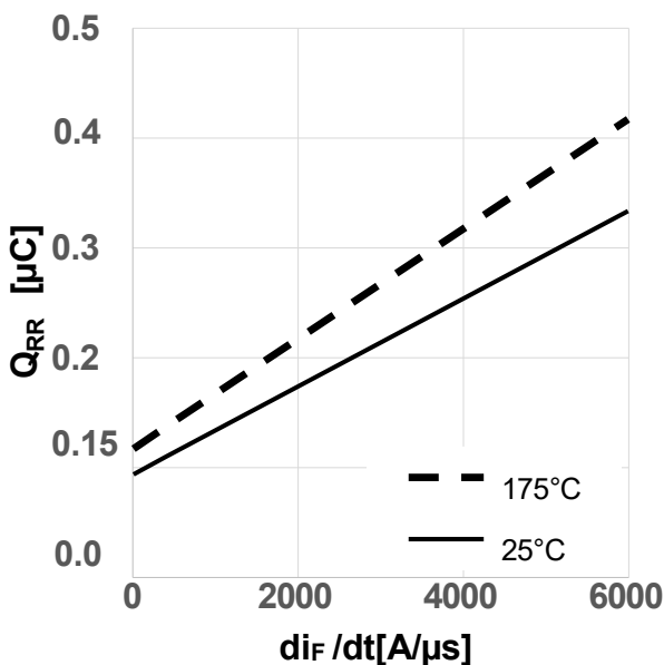
图 19 典型的反向恢复电荷随二极管电流斜率变化关系 (Q_{rr} = f(di_i/dt), V_{DD} = 800V, V_{GS} = 0V/18V, I_D = 8.5A, \text{独立负载, 测试电路见图 E, } V_{GS} = 0V \text{ 时的体二极管})
