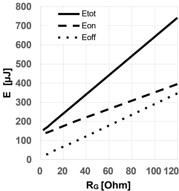
图 17 典型开关能量损耗随栅极电阻变化关系 (E = f(R_{G,ext}), V_{DD} = 800V, V_{GS} = 0V/18V, I_D = 8.5A, T_{vj} = 175^\circ C, \text{独立负载, 测试电路见图 E, 二极管: } V_{GS} = 0V) \text{ 时的体二极管}
