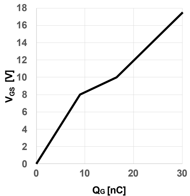
典型栅极电荷
