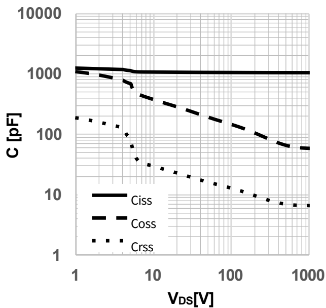
图 11 典型电容随漏源电压变化关系 ( C = f(V_{DS}) , V_{GS} = 0V , f = 1MHz )
