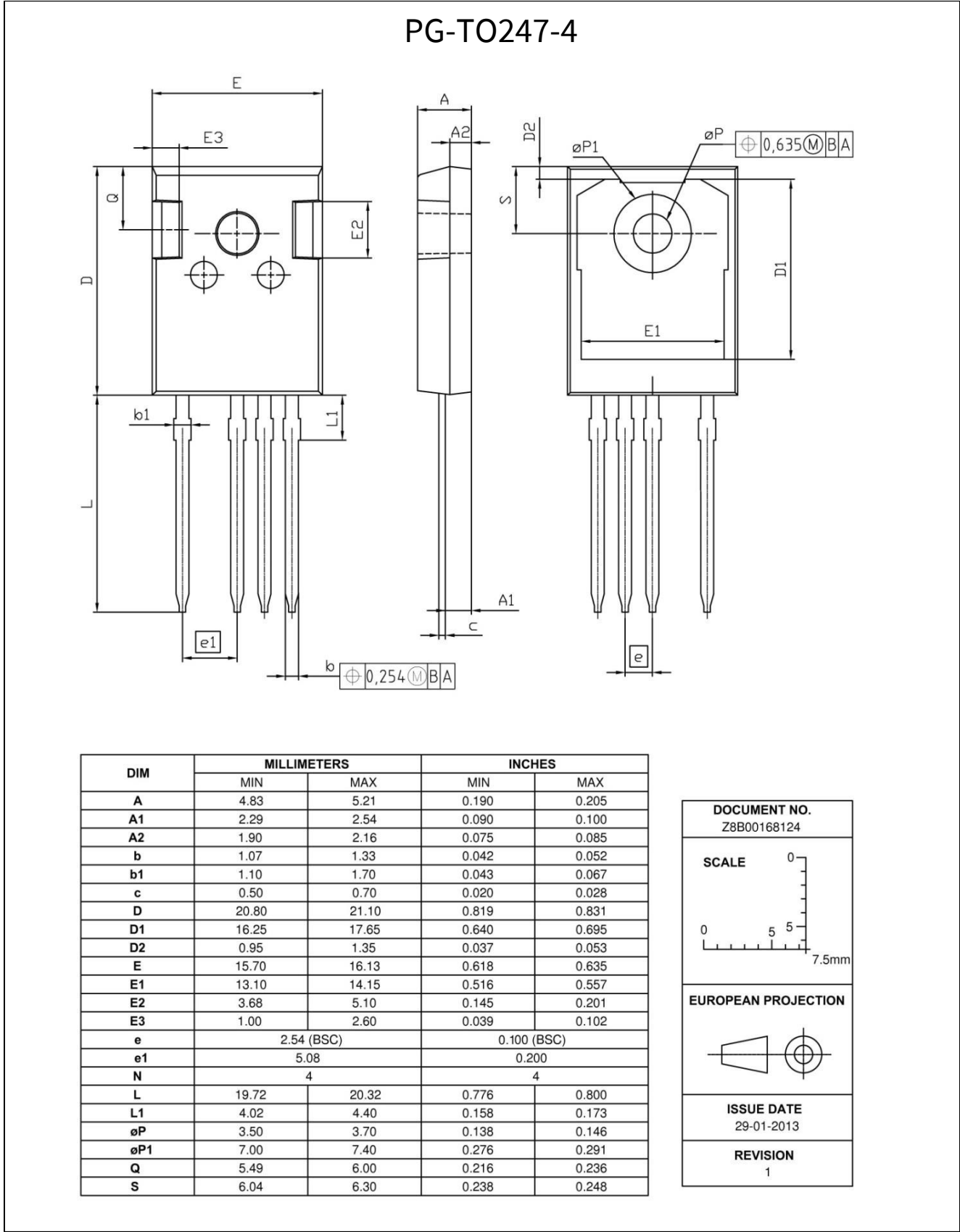
图 22 封装图
