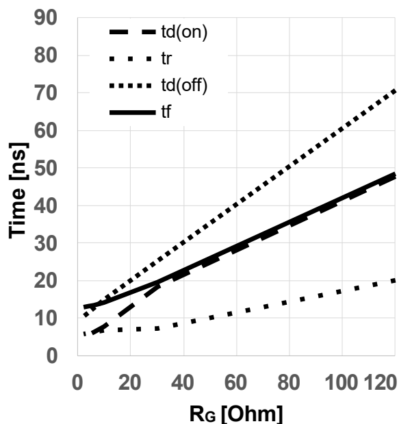
图 18 典型开关时间随栅极电阻变化关系 (t = f(R_{G,ext}), V_{DD} = 800V, V_{GS} = 0V/18V, I_D = 6A, T_{vj} = 175^\circ C, \text{独立负载, 测试电路见图 E, 二极管: } V_{GS} = 0V \text{ 时的体二极管})
