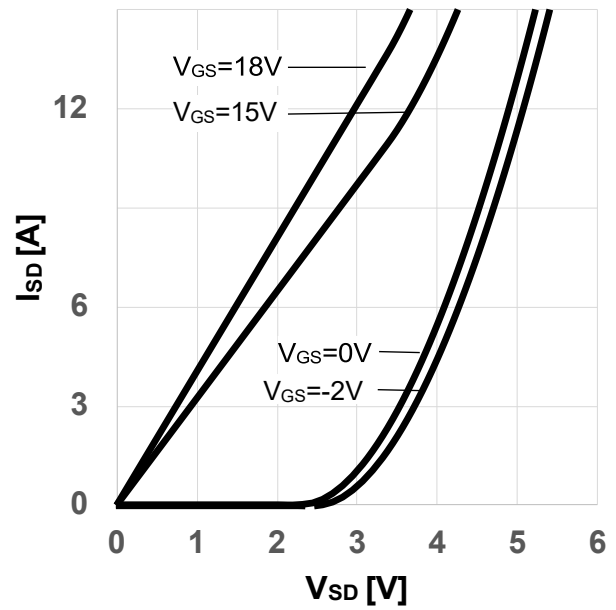
图 14 典型体二极管正向电流随正向电压变化关系， V_{GS} 为参数
