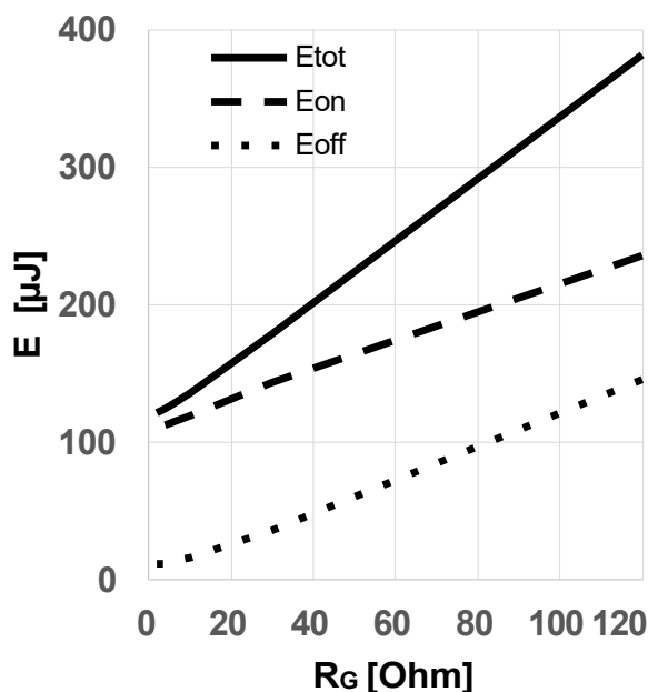
图 17 典型开关能量损耗随栅极电阻变化关系 (E = f(R_{G,ext}), V_{DD} = 800V, V_{GS} = 0V/18V, I_D = 6A, T_{vj} = 175^\circ C, \text{独立负载, 测试电路见图 E, 二极管: } V_{GS} = 0V \text{ 时的体二极管})
