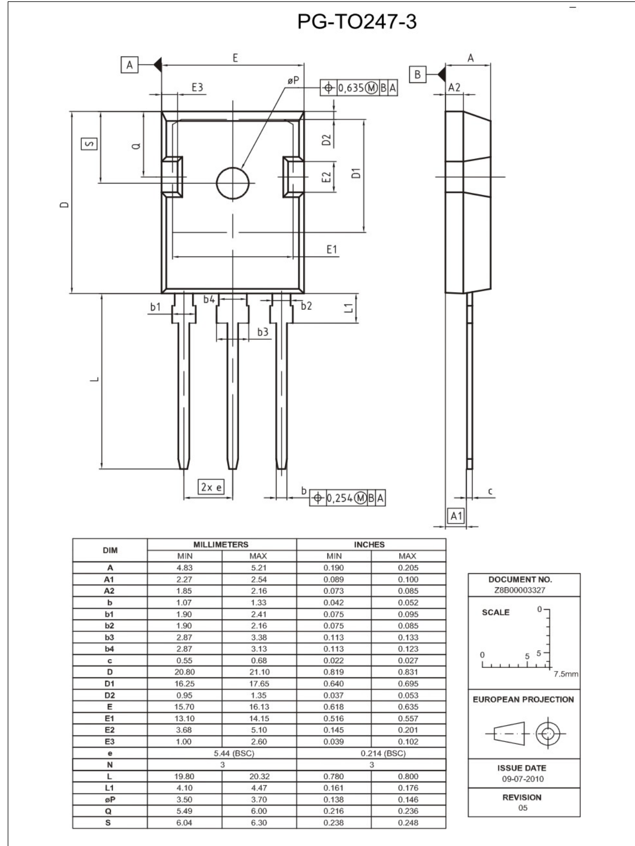
图 22 封装图
