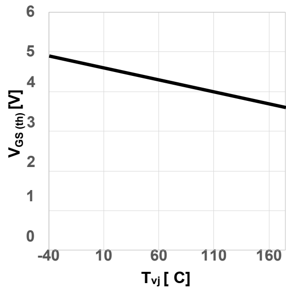
图 6 典型栅极-源极阈值电压与结温的函数关
