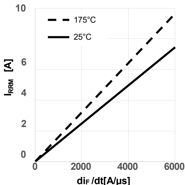
图 20 典型反向恢复电流随二极管电流斜率变化关系 (I_{rrm} = f(di_f/dt), V_{DD} = 800V, V_{GS} = 0V/18V, I_D = 6A, \text{独立负载, 测试电路如图 E 所示, 体二极管在 } V_{GS} = 0V \text{ 时})
