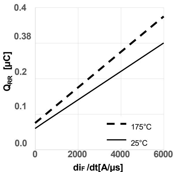
图 19 典型的反向恢复电荷随二极管电流斜率变化关系 (Q_{rr} = f(di_f/dt), V_{DD} = 800V, V_{GS} = 0V/18V, I_D = 6A, \text{独立负载, 测试电路见图 E, } V_{GS} = 0V \text{ 时的体二极管})
