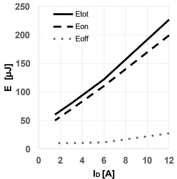
图 16 典型开关能量损耗随漏源电流变化关系
