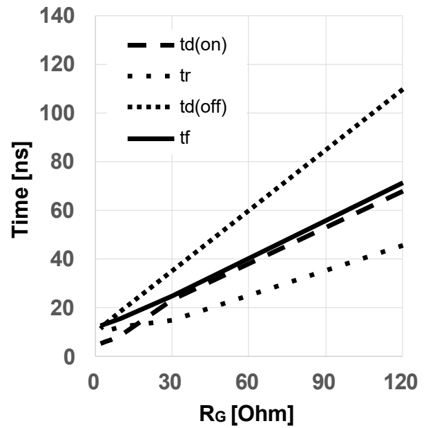
图 18 典型开关时间随栅极电阻变化关系 (t = f(R_{G,ext}), V_{DD} = 800V, V_{GS} = 0V/18V, I_D = 8.5A, T_{vj} = 175^\circ C, \text{独立负载, 测试电路见图 E, 二极管: } V_{GS} = 0V) \text{ 时的体二极管}
