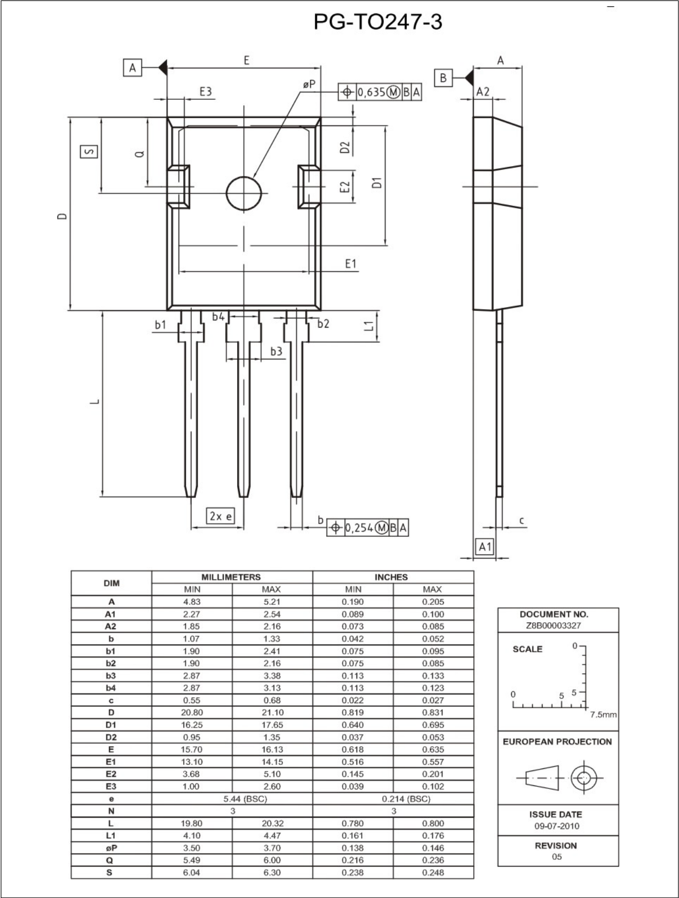
图 22 封装图
