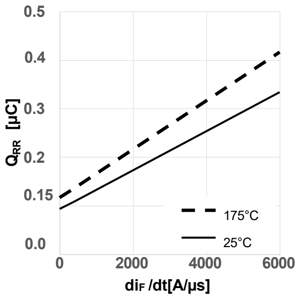
图 19 典型的反向恢复电荷随二极管电流斜率变化关系 (Q_{rr} = f(di_F/dt), V_{DD} = 800V, V_{GS} = 0V/18V, I_D = 8.5A, \text{独立负载, 测试电路见图 E, } V_{GS} = 0V \text{ 时的体二极管})
