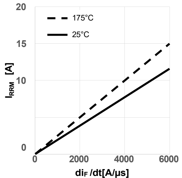
图 20 典型反向恢复电流随二极管电流斜率变化关系 (I_{rrm} = f(di_F/dt), V_{DD} = 800V, V_{GS} = 0V/18V, I_D = 8.5A, \text{独立负载, 测试电路如图 E 所示, 体二极管在 } V_{GS} = 0V \text{ 时})
