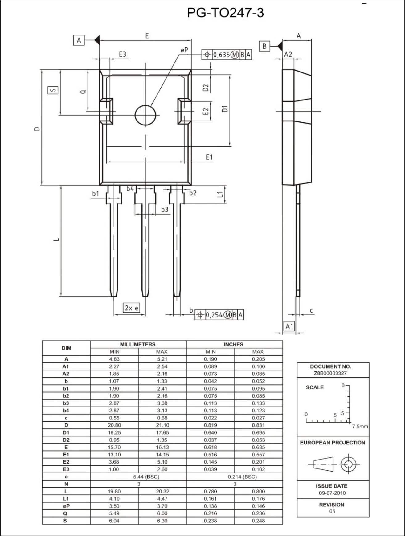
图 22 封装图
