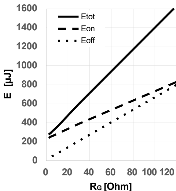
图 17 典型开关能量损耗随栅极电阻变化关系 (E = f(R_{G,ext}), V_{DD} = 800V, V_{GS} = 0V/18V, I_D = 13A, T_{vj} = 175^\circ C, \text{独立负载, 测试电路见图 E, 二极管: } V_{GS} = 0V \text{ 时的体二极管})
