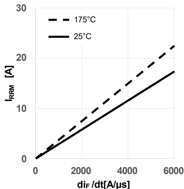
图 20 典型反向恢复电流随二极管电流斜率变化关系 (I_{rrm} = f(di_F/dt), V_{DD} = 800V, V_{GS} = 0V/18V, I_D = 13A, \text{独立负载, 测试电路如图 E 所示, 体二极管在 } V_{GS} = 0V \text{ 时})
