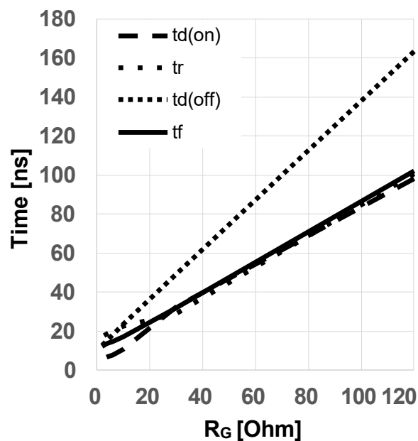
图 18 典型开关时间随栅极电阻变化关系 (t = f(R_{G,ext}), V_{DD} = 800V, V_{GS} = 0V/18V, I_D = 13A, T_{vj} = 175^\circ C, \text{独立负载, 测试电路见图 E, 二极管: } V_{GS} = 0V \text{ 时的体二极管})
