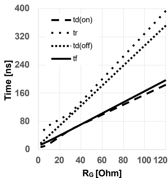
图 18 典型开关时间随栅极电阻变化关系 (t = f(R_{G,ext}), V_{DD} = 800V, V_{GS} = 0V/18V, I_D = 25A, T_{vj} = 175^\circ C, \text{独立负载, 测试电路见图 E, 二极管: } V_{GS} = 0V) \text{ 时的体二极管}
