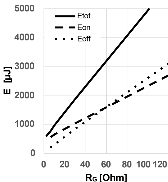
图 17 典型开关能量损耗随栅极电阻变化关系 (E = f(R_{G,ext}), V_{DD} = 800V, V_{GS} = 0V/18V, I_D = 25A, T_{vj} = 175^\circ C, \text{独立负载, 测试电路见图 E, 二极管: } V_{GS} = 0V) \text{ 时的体二极管}
