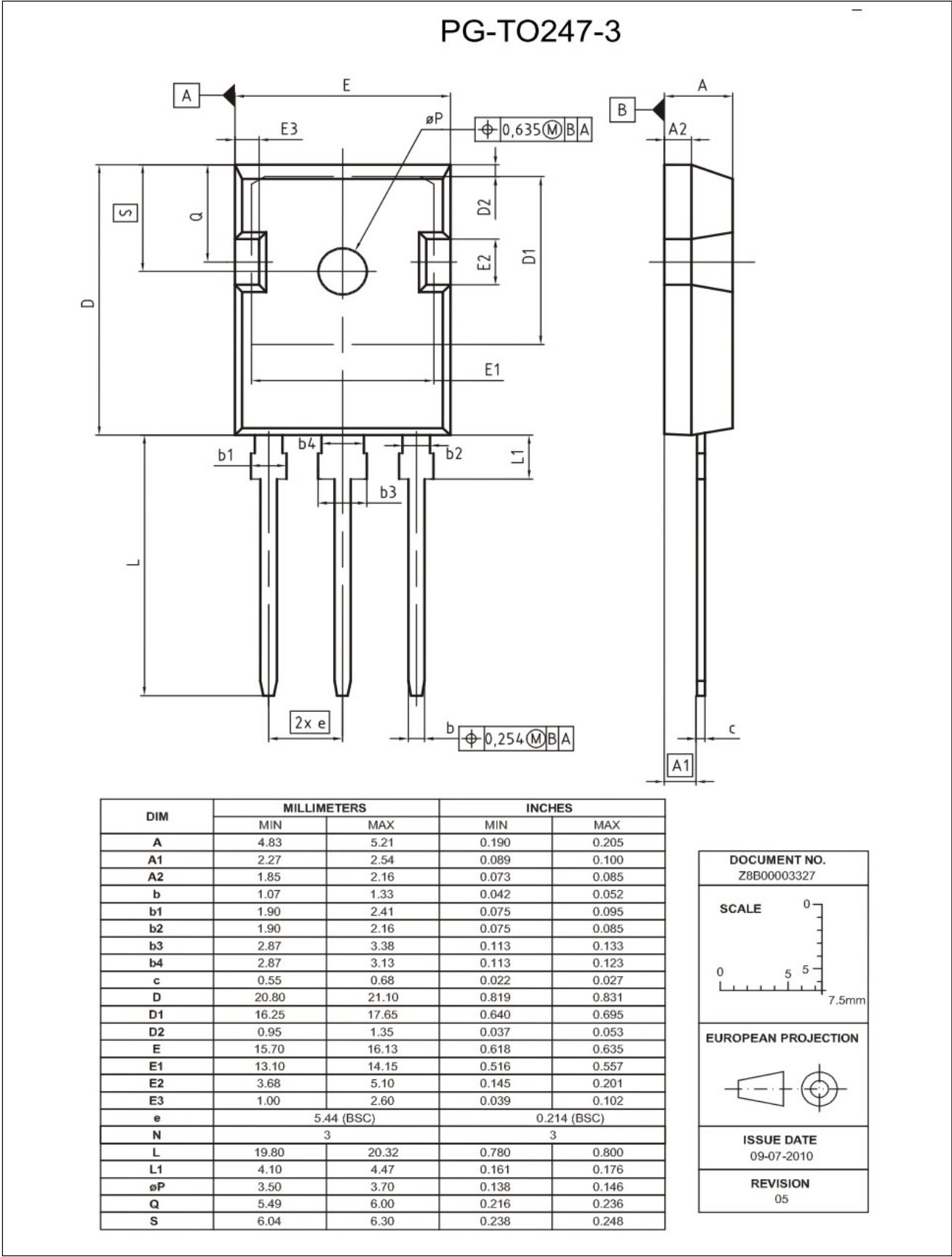
图 22 封装图
