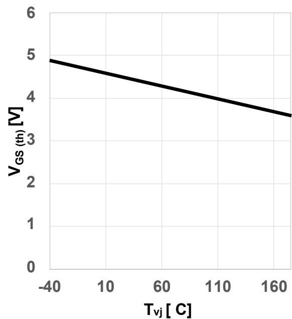
图 6: 典型栅极-源极阈值电压随结温变化关系
