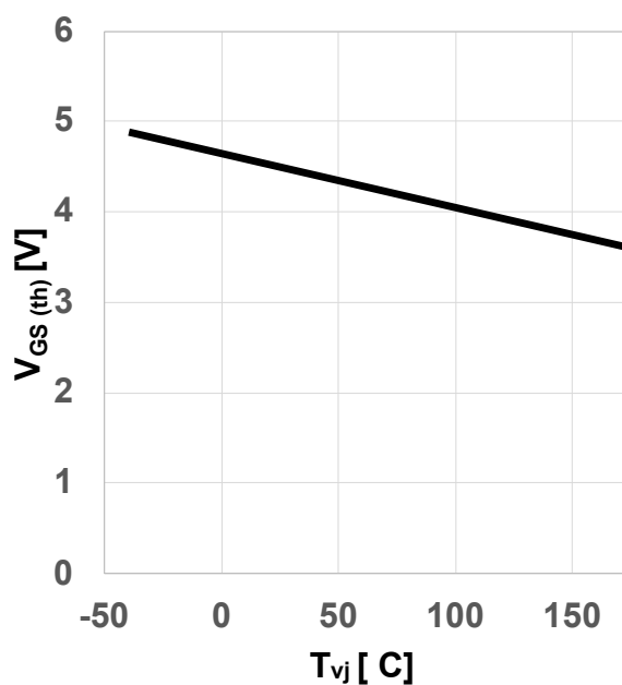
图 6 典型栅极-源极阈值电压与结温的函数关系
