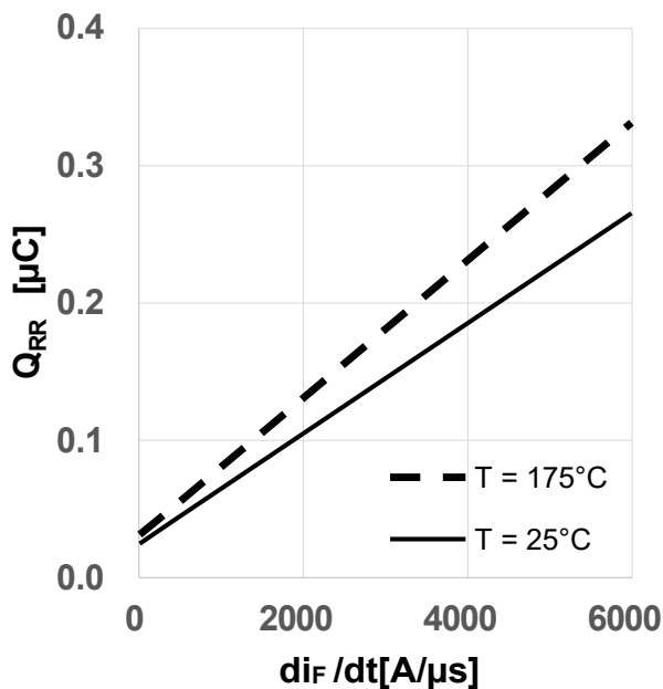
图 19 典型的反向恢复电荷随二极管电流斜率变化关系 (Q_{rr} = f(di_F/dt), V_{DD} = 800V, V_{GS} = 0V/18V, I_D = 2A, \text{独立负载, 测试电路见图 E, } V_{GS} = 0V \text{ 时的体二极管})
