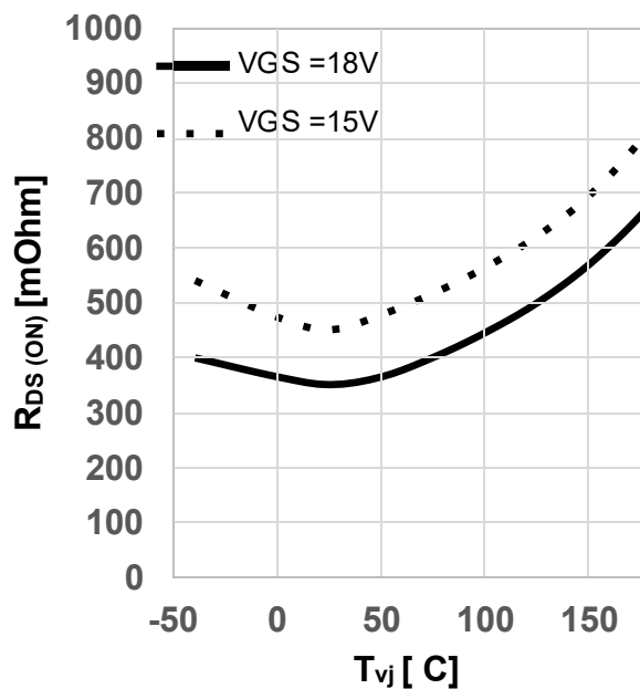
图 9 典型导通电阻随结温变化关系
