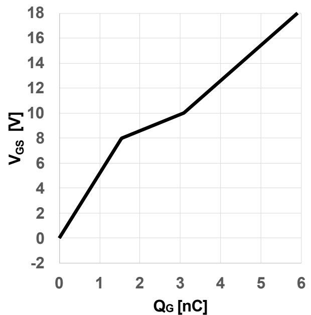
图 10 典型栅极电荷
