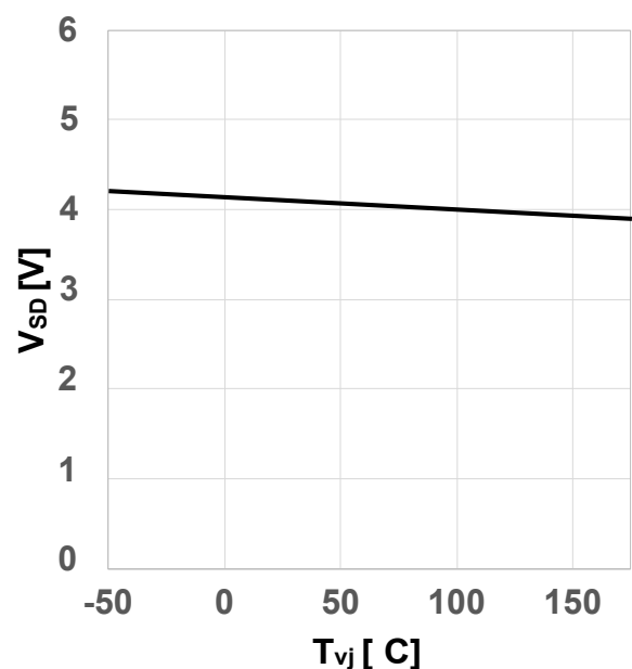
图 12 典型体二极管正向电压随结温变化
