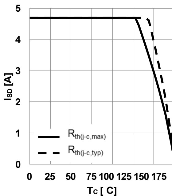
图4 最大源漏电流随壳温 (受限于接合线) 变化关系 ( I_{SD} = f(T_c) , V_{GS} = 0V )
