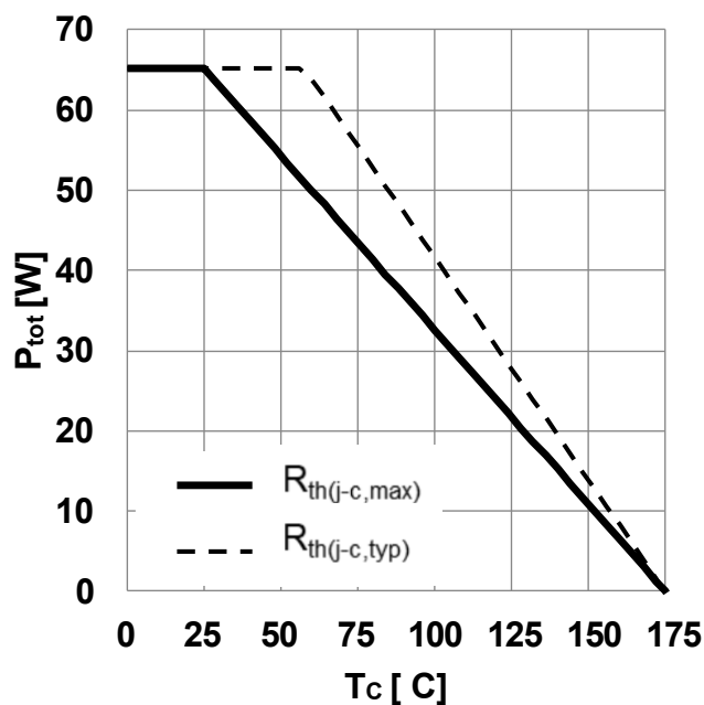
图2 功率耗散随壳温 (受限于接合线) 变化关系 ( P_{tot} = f(T_c) )
