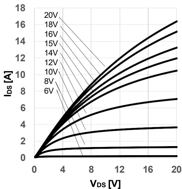
图 8 典型输出特性, V_{GS} 为参数
