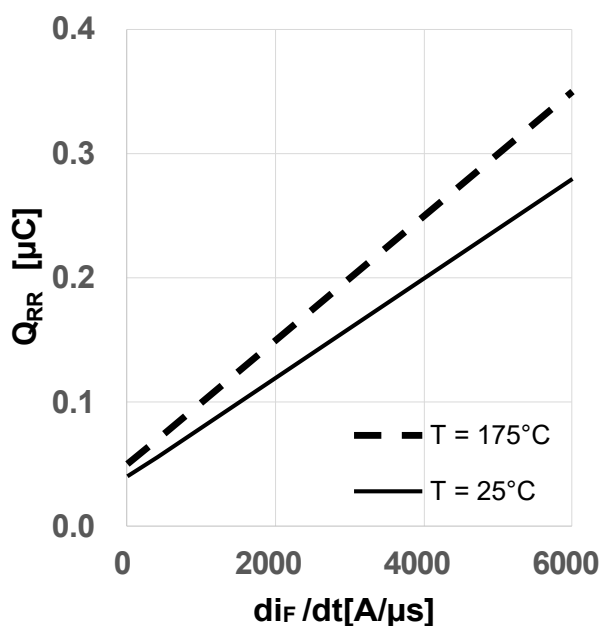
图 19 典型的反向恢复电荷随二极管电流斜率变化关系 (Q_{rr} = f(di/dt), V_{DD} = 800V, V_{GS} = 0V/18V, I_D = 4A, \text{独立负载, 测试电路见图 E, } V_{GS} = 0V \text{ 时的体二极管})
