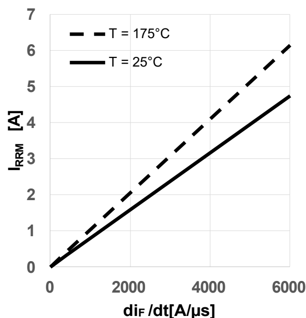
图 20 典型反向恢复电流随二极管电流斜率变化关系 (I_{rrm} = f(di/dt), V_{DD} = 800V, V_{GS} = 0V/18V, I_D = 4A, \text{独立负载, 测试电路如图 E 所示, 体二极管在 } V_{GS} = 0V \text{ 时})
