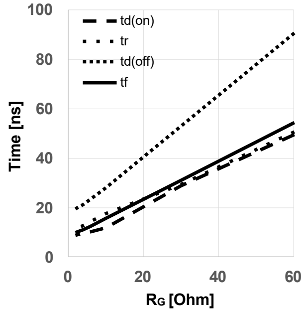
图 18 典型开关时间随栅极电阻变化关系 (t = f(R_{G,ext}), V_{DD} = 800V, V_{GS} = 0V/18V, I_D = 13A, T_{vj} = 175^\circ C, \text{独立负载, 测试电路见图 E, 二极管: } V_{GS} = 0V \text{ 时的体二极管})
