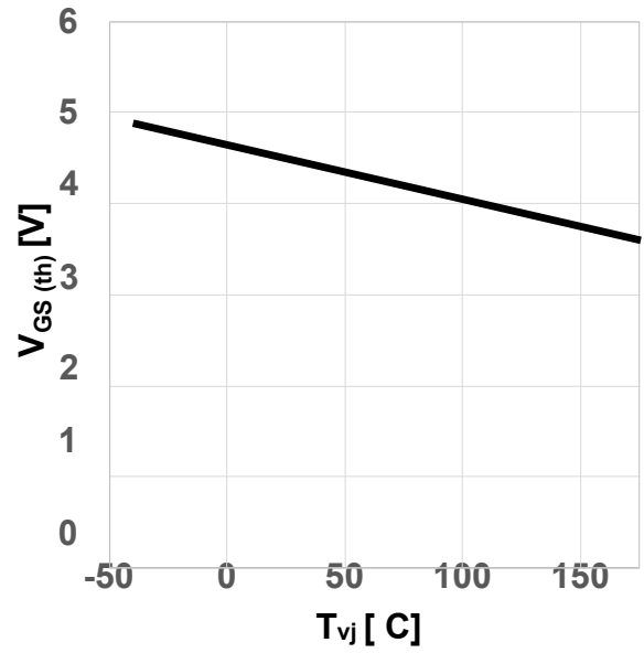
图 6 典型栅极-源极阈值电压与结温的函数关系
