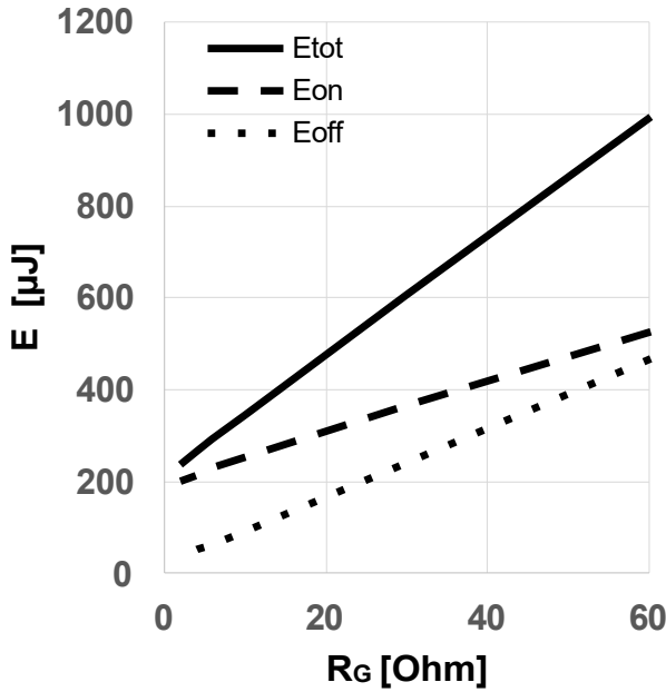
图 17 典型开关能量损耗随栅极电阻变化关系 (E = f(R_{G,ext}), V_{DD} = 800V, V_{GS} = 0V/18V, I_D = 13A, T_{vj} = 175^\circ C, \text{独立负载, 测试电路见图 E, 二极管: } V_{GS} = 0V \text{ 时的体二极管})
