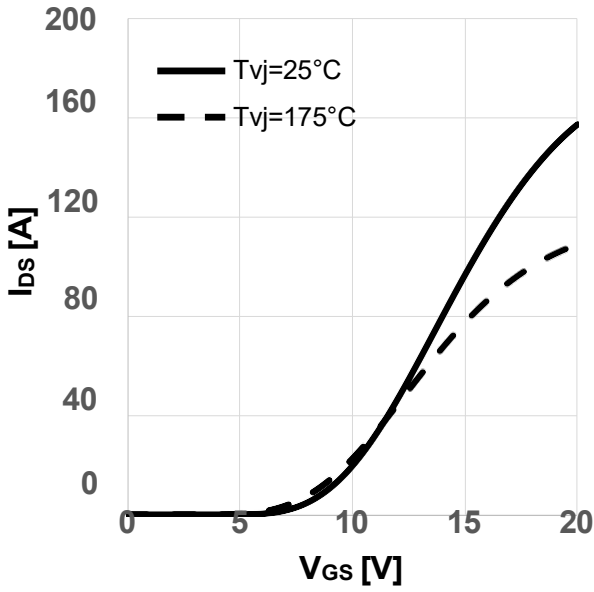
图 5 典型传输特性
