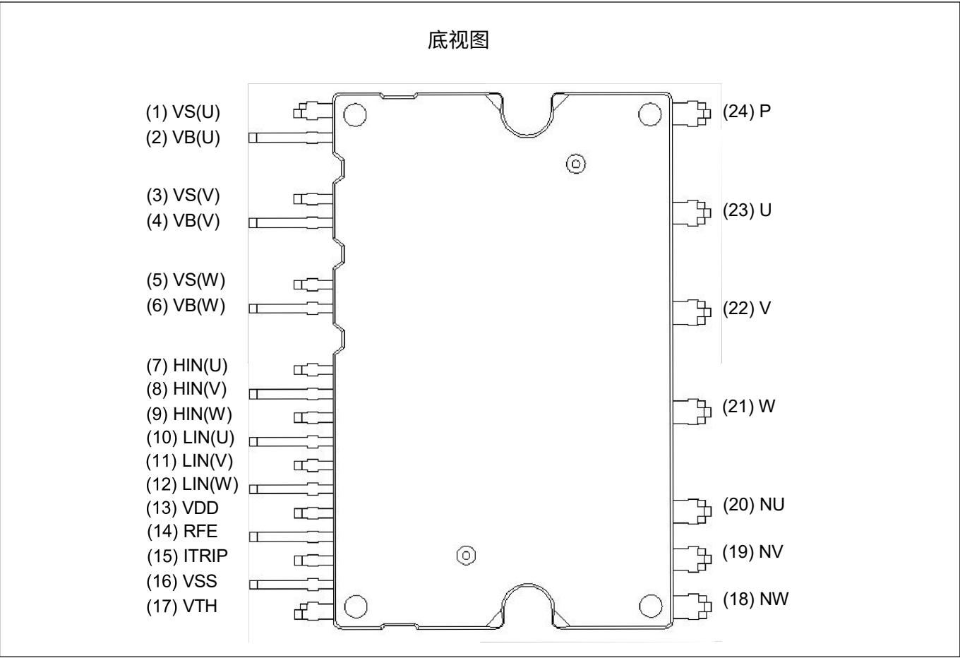
图 2 模块引脚分布表
