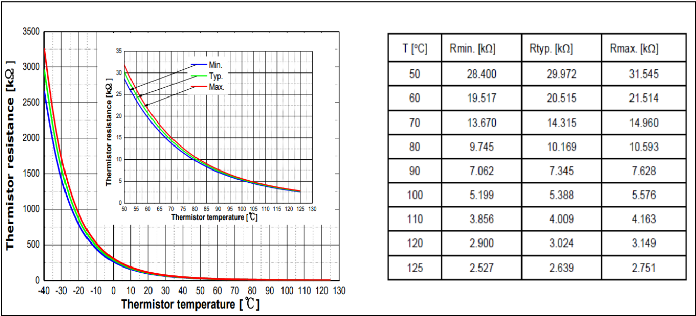
图6 热敏电阻阻值-温度曲线及表格 (更多信息请参考应用笔记‘AN2019-16 CIPOS™ Maxi IM818应用笔记’)
