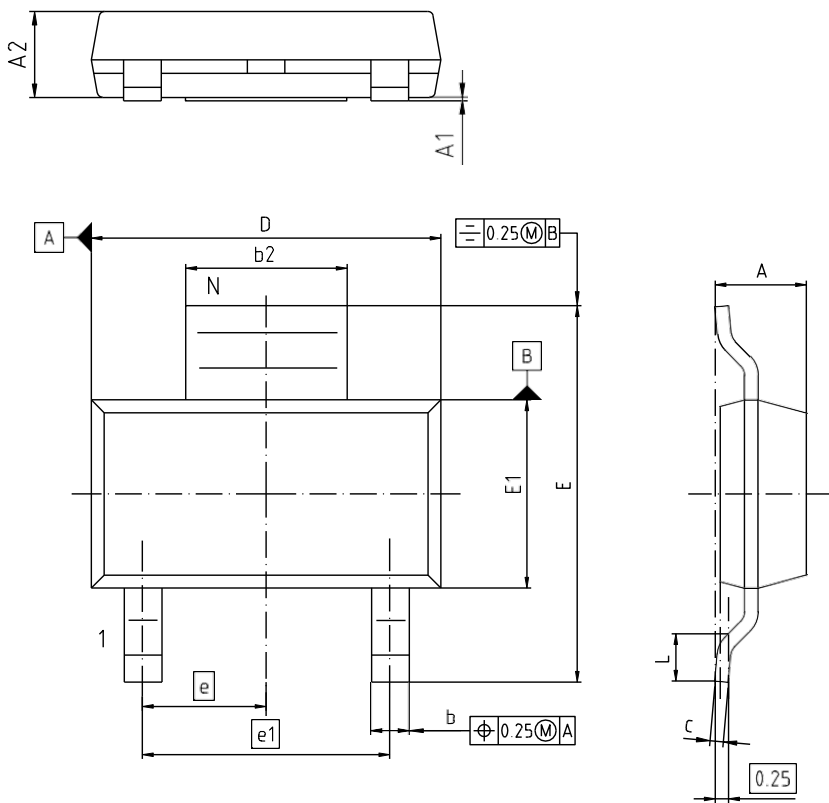
PG-SOT223-3
