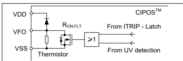
图 5 VFO 引脚内部电路
