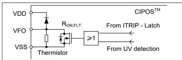
图 5 VFO 引脚内部电路
