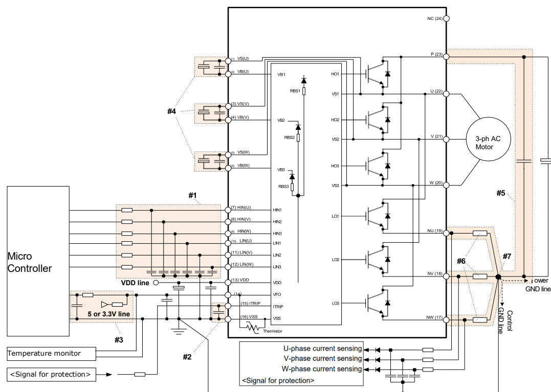
图9 典型应用电路
