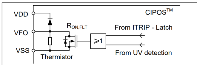
图 5 VFO 引脚内部电路
