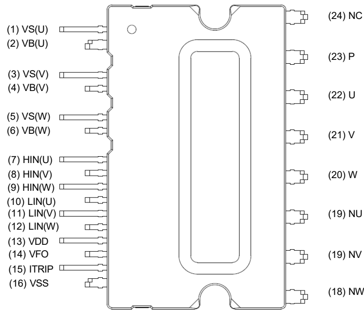
底视图
