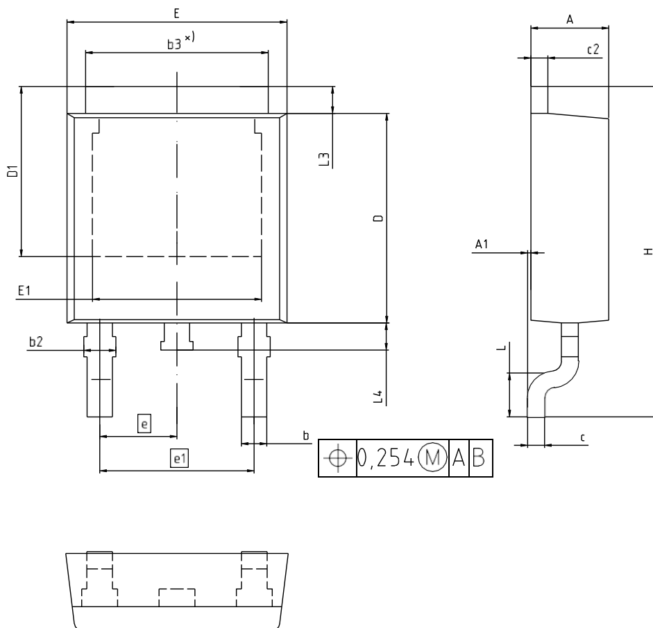
封装图 PG-TO252-3
