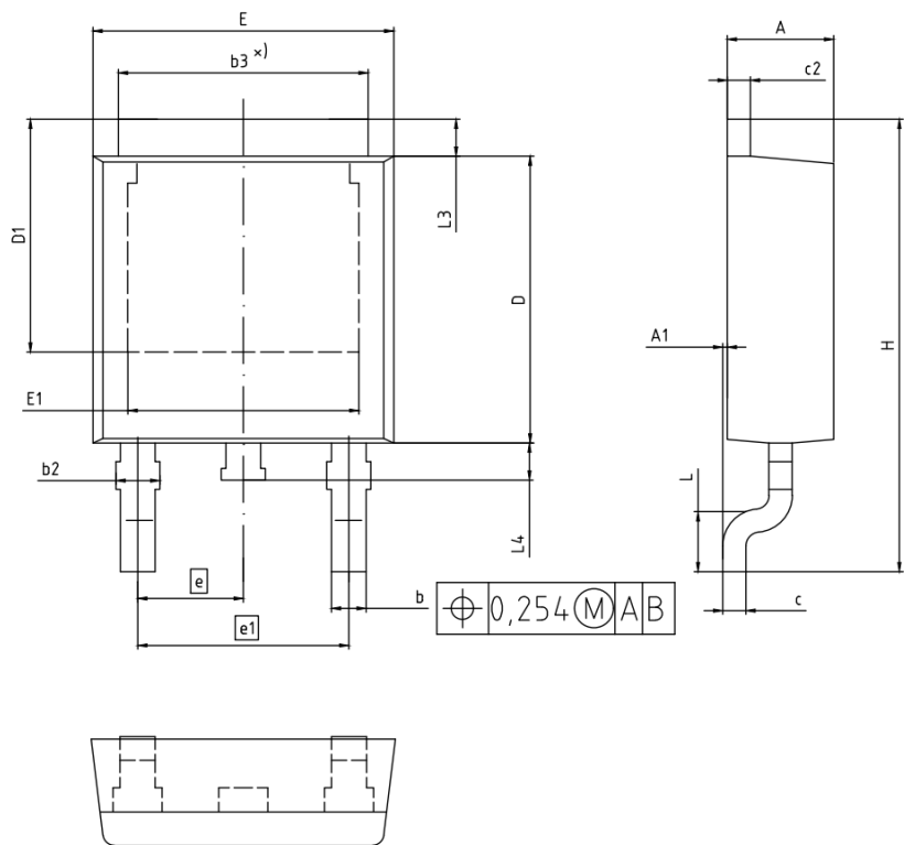
封装图 PG-TO252-3
