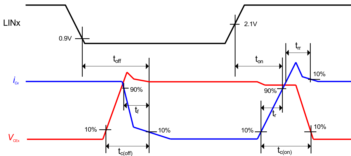
图 10 开关时间定义
