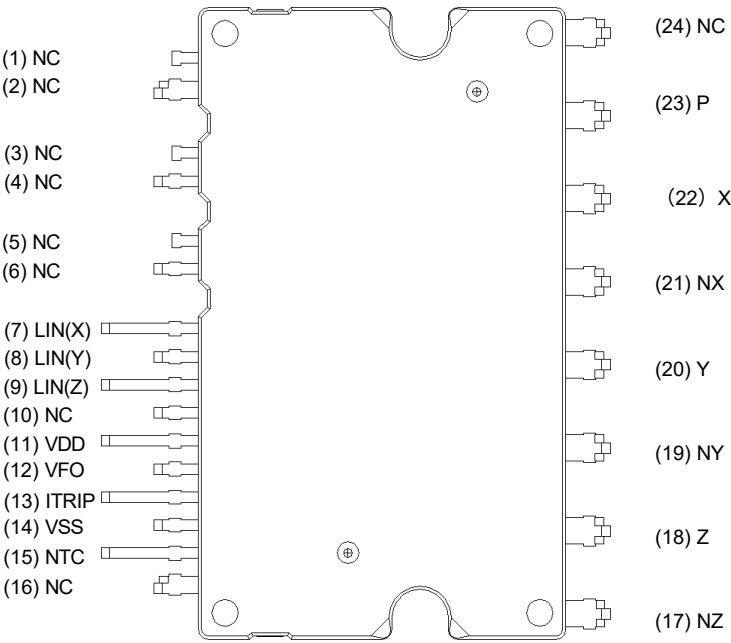
底视图
