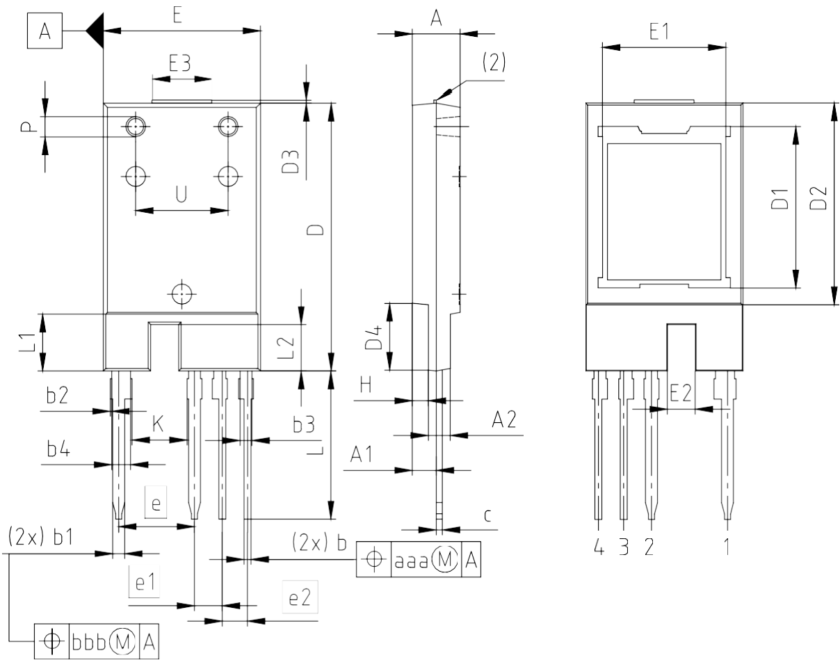
PG-TO247-4-PLUS-NT14
