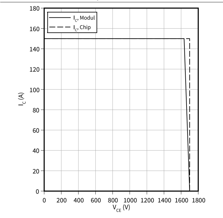
逆バイアス安全動作領域 (RBSOA), IGBT- インバータ I_C = f(V_{CE}) R_{Goff} = 1\ \Omega , V_{GE} = \pm 15\text{ V} , T_{vj} = 150\text{ }^\circ\text{C}
