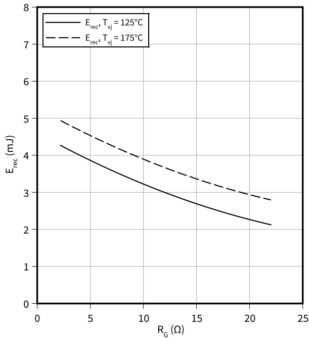
スイッチング損失 (typical), Diode、インバータ E_{rec} = f(R_G) V_{CE} = 600\ \text{V} , I_F = 75\ \text{A}
