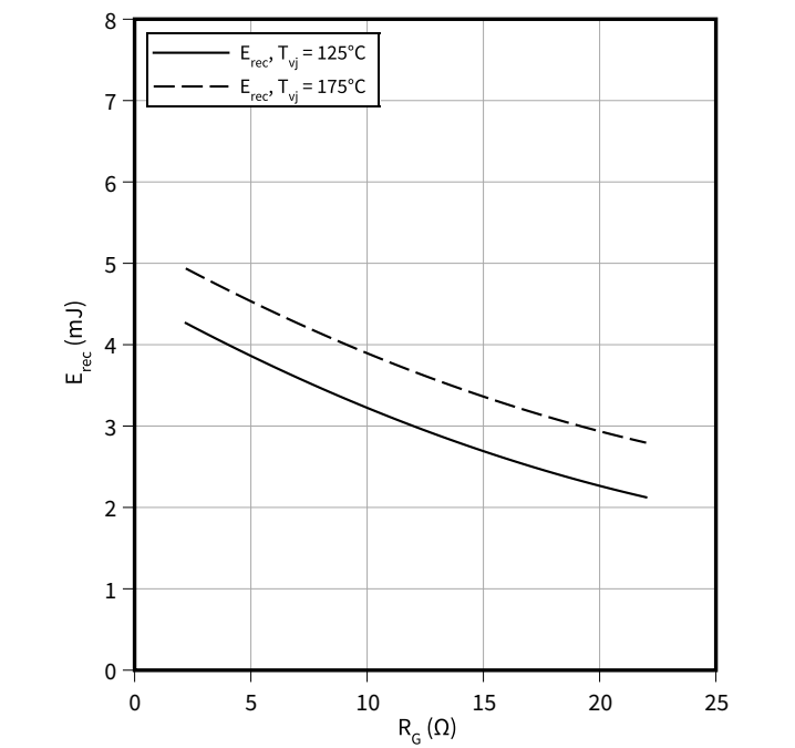
开关损耗（典型），二极管,逆变器 E_{rec} = f(R_G) V_{CE} = 600 V, I_F = 75 A
