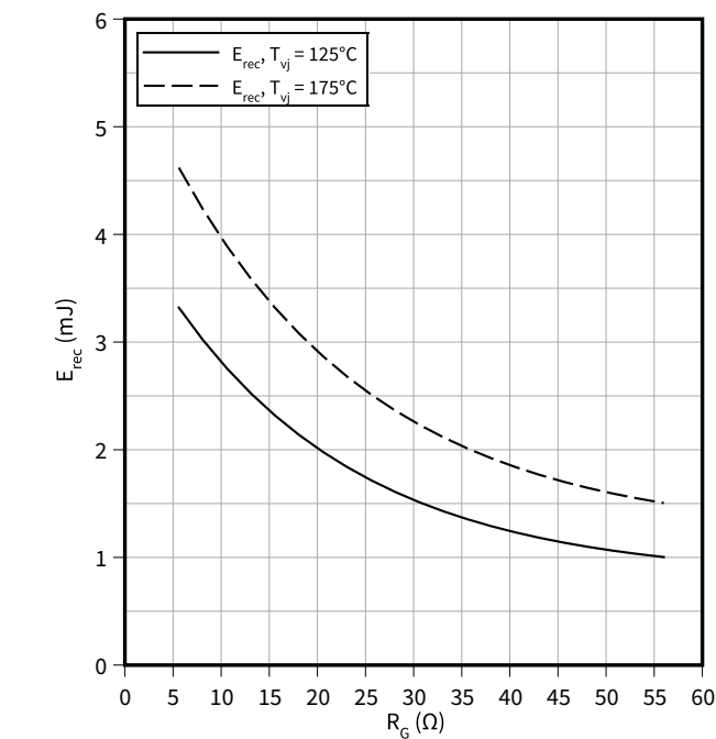
开关损耗（典型），二极管，逆变器 E_{rec} = f(R_G) I_F = 75 \text{ A} , V_R = 600 \text{ V}
