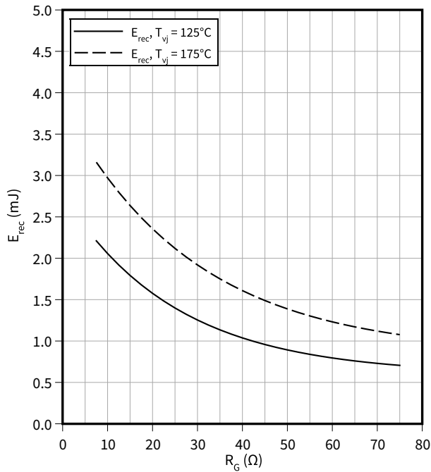
スイッチング損失 (typical), Diode、インバータ E_{rec} = f(R_G) I_F = 50\ \text{A} , V_R = 600\ \text{V}
