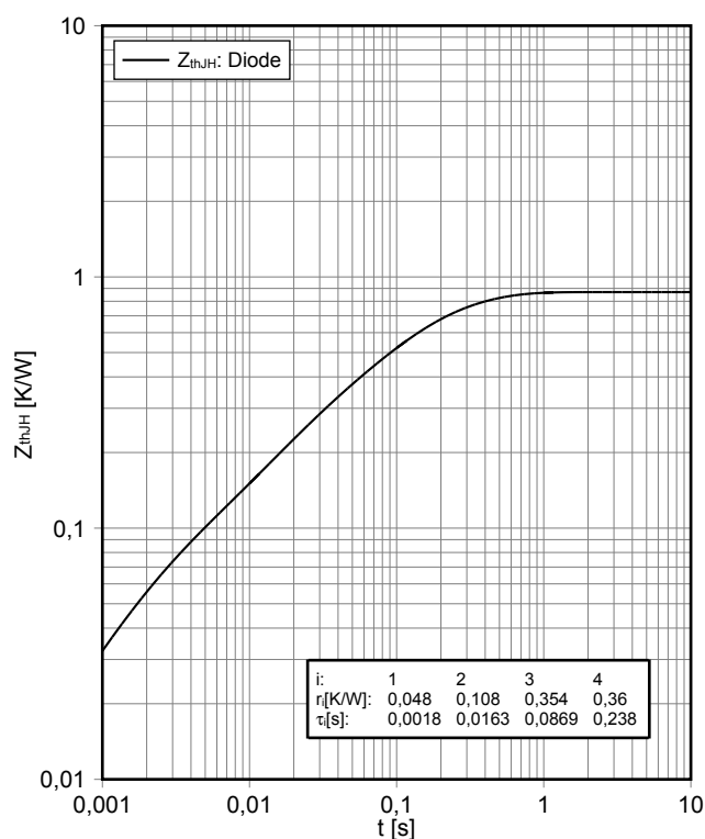
過渡熱インピーダンス バイパスダイオード transient thermal impedance Bypass-Diode Z_{thJH} = f(t)
