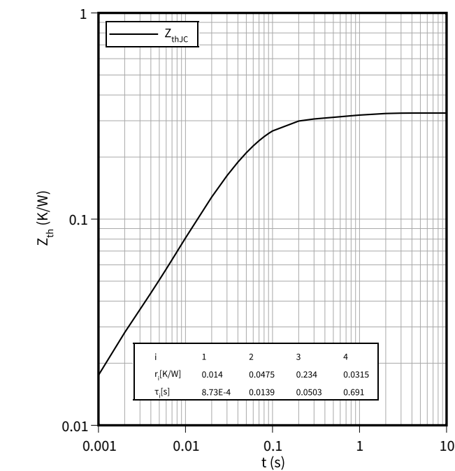
瞬态热阻抗, 二极管, 制动-斩波器 Z_{th} = f(t)
