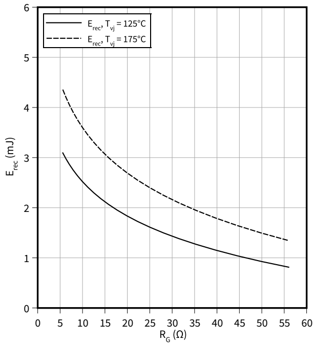
スイッチング損失 (typical), Diode、インバータ E_{rec} = f(R_G) I_F = 75\ \text{A} , V_R = 600\ \text{V}
