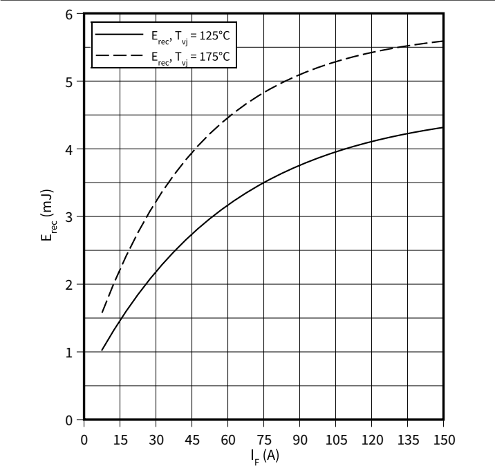
开关损耗（典型), 二极管, 逆变器
